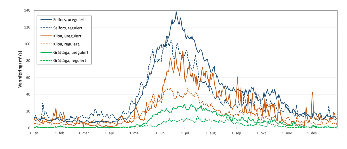
Figur 2. Gjenomsnittlig vannføring (døgnsnitt) gjennom året i Beiarelva før og etter reguleringen i Gråttåga (1975-1999), ved Klipa (1989-2014) og ved Selfors i nedre del av elven (1916-2014). Data fra NVE.
