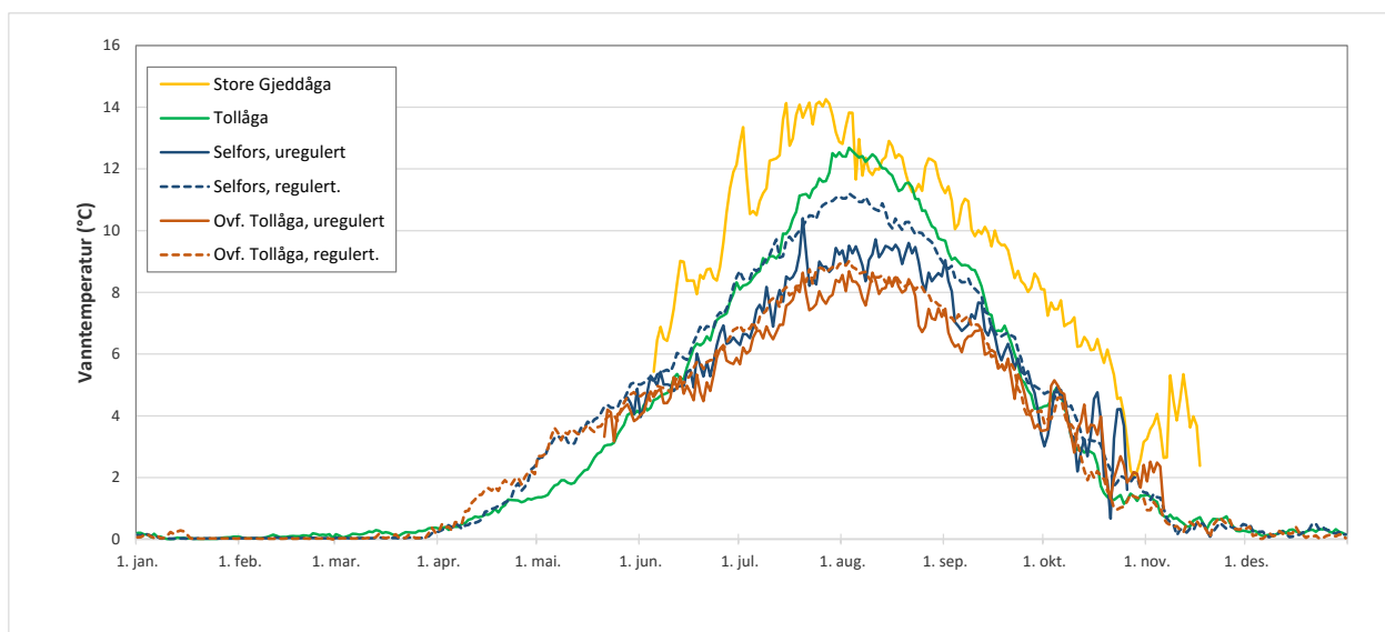
Figur 4. Gjennomsnittlig vannføring (døgnsnitt) gjennom året i Store Gjeddåga (1999-2000, bare sommer), Tollåga (1983-2014, bare sommer før 2005), Beiareelva før og etter reguleringen ovenfor Tollåga (1984-2003 og 2010-2015, bare sommer før 2001), og ved Selfors i nedre del av elven (1985-2015, bare sommer før 2007). Data fra NVE.
