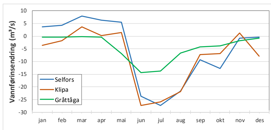
Figur 3. Gjenomsnittlig vannføringsendring (månedssnitt) etter reguleringen i Gråttåga (1975-1999), ved Klipa (1989-2014), og ved Selfors i nedre del av elven (1916-2014). Data fra NVE.
