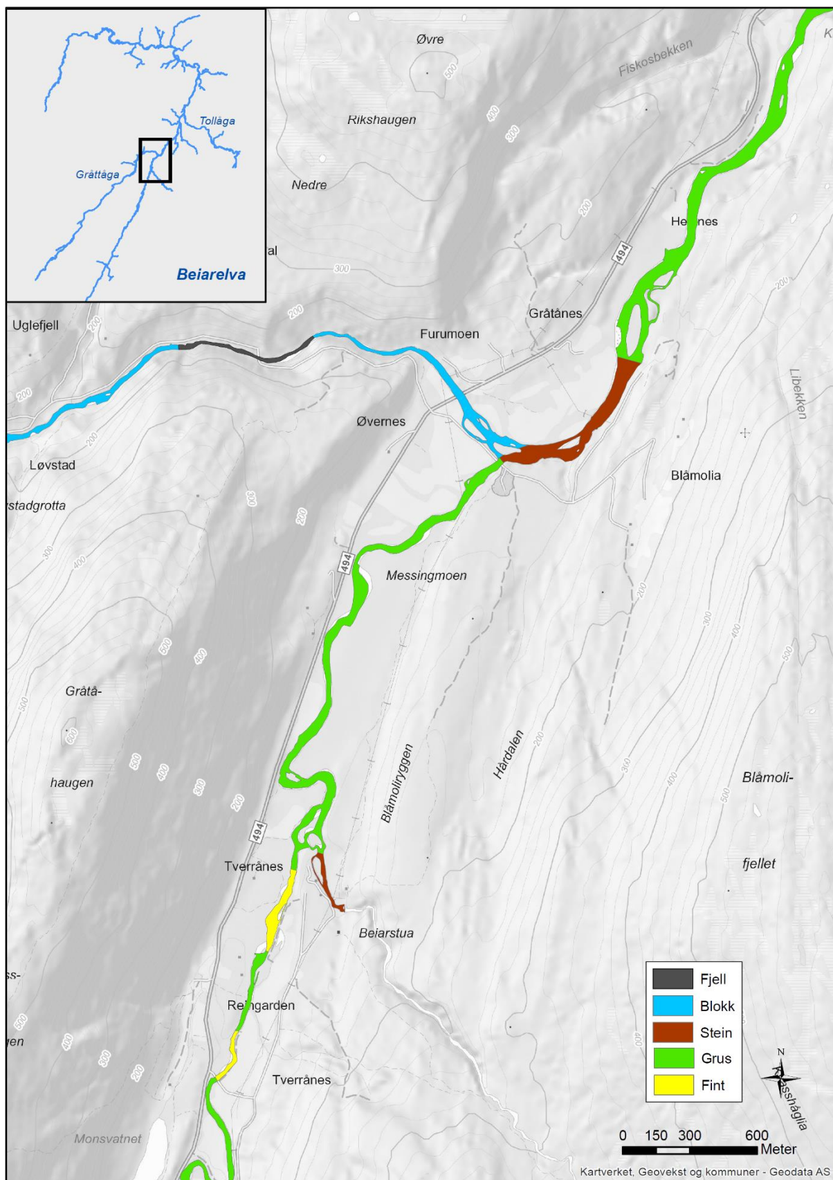
Figur 20. Fordeling av dominerende substrattyper på ikke-anadrom del av Beiarelva (Rydeng - Klipa).
