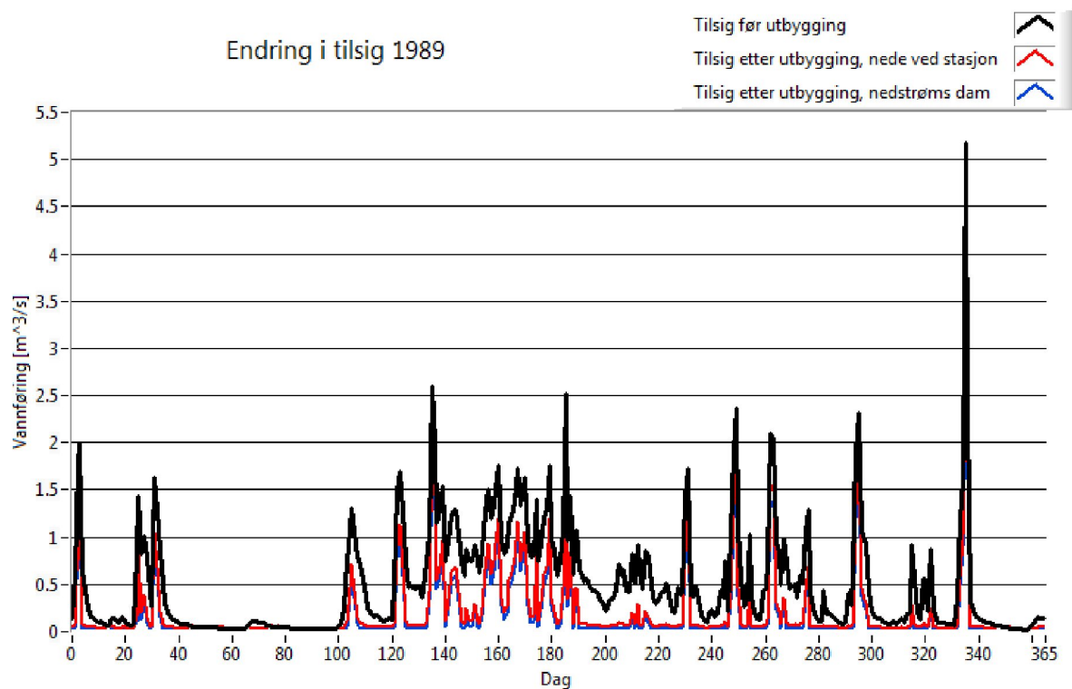
Figur 8. Plott som viser vannføringsvariasjoner i et vått (1989) år (før og etter utbygging). 18
