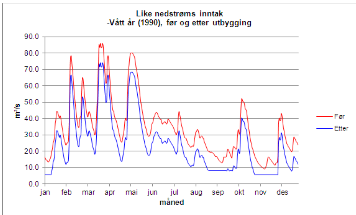
Plott som viser vassføringsvariasjonar i eit vått (1990) år (før og etter utbygging)
