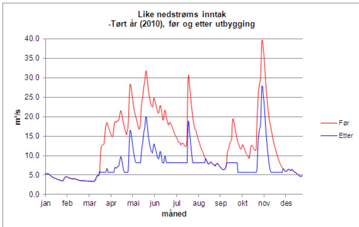
Plott som viser vassføringsvariasjonar i eit tørt (2010) år (før og etter utbygging)
