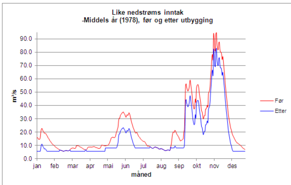
Plott som viser vassføringsvariasjonar i eit middels (1978) år (før og etter utbygging)
