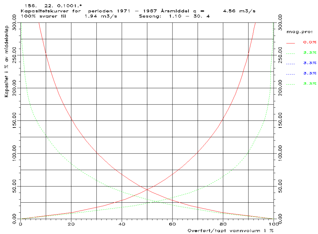
Figur 10. Varighetskurve for vintersesongen (1/10 - 30/4).
