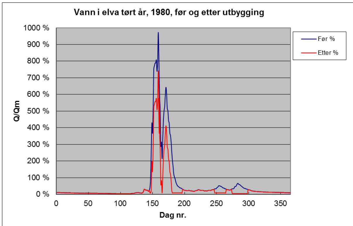
Plot 2: Viser vannføringsvariasjoner i et tørt (1980) år (før og etter utbygging).
