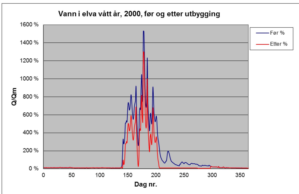
Plot 4: Viser vannføringsvariasjoner i et vått (2000) år (før og etter utbygging).
