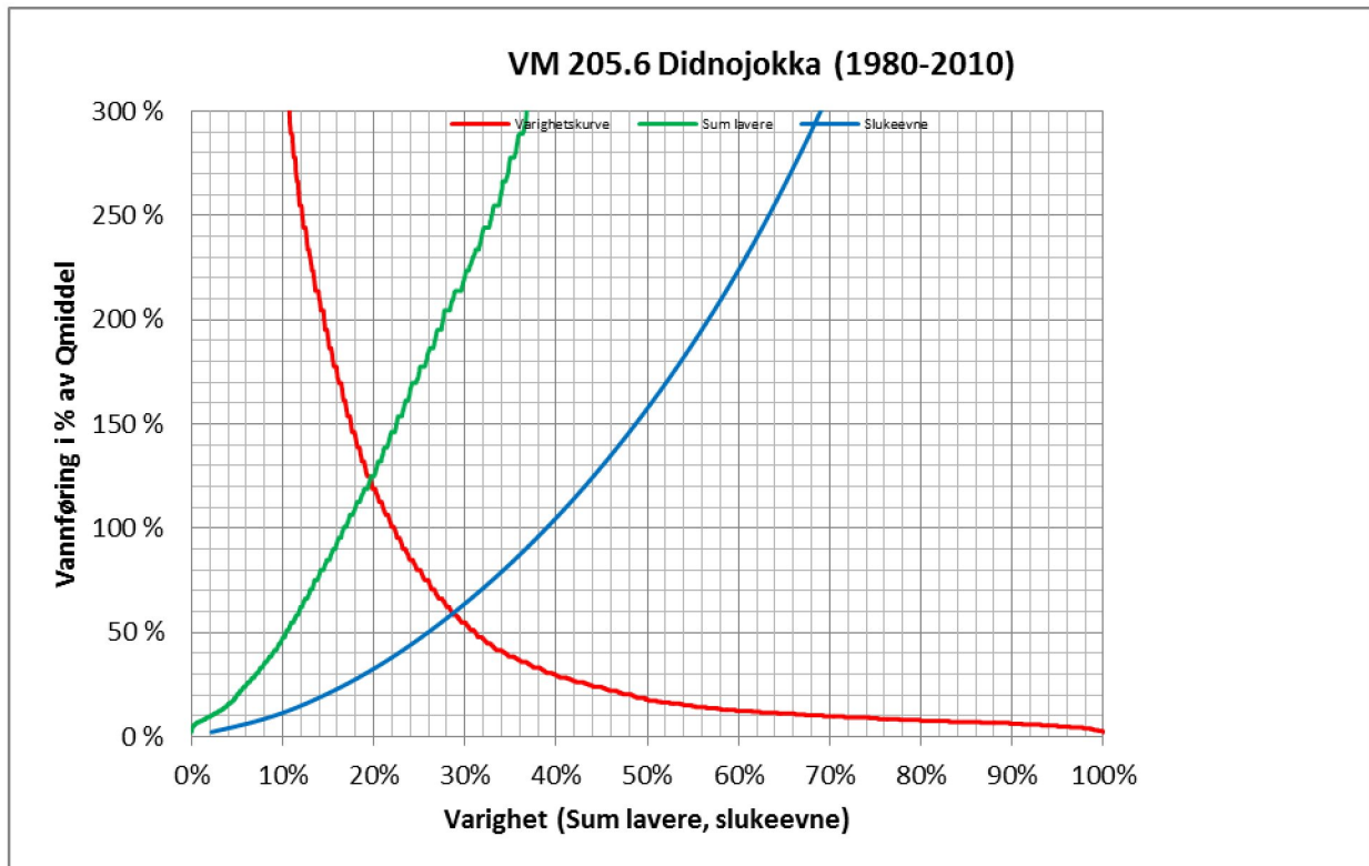
Plot 1: Varighetskurve, kurve for flomtap og for tap av vann i lavvannsperioden (år).
