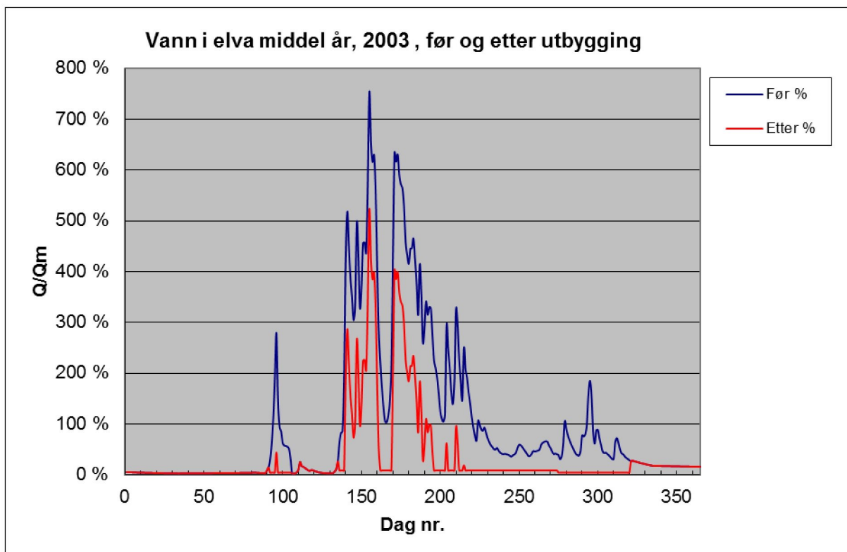
Plot 3: Viser vannføringsvariasjoner i et middel (2003) år (før og etter utbygging).
