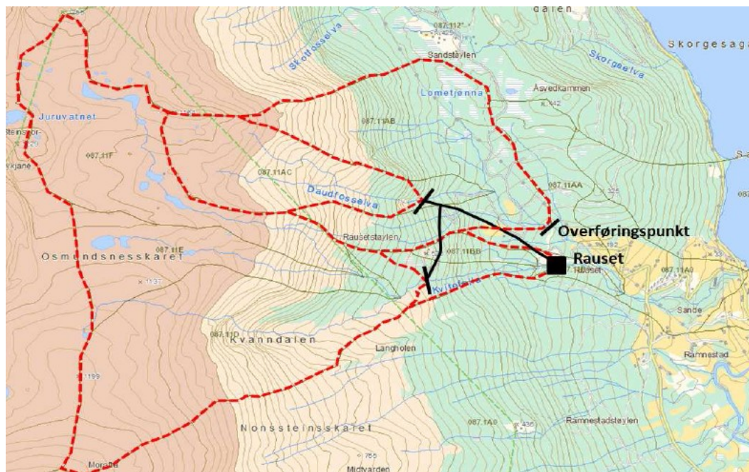
Nedbørsfelt og restfelt. Overføringspunkt til Kvitfella kraftverk.
