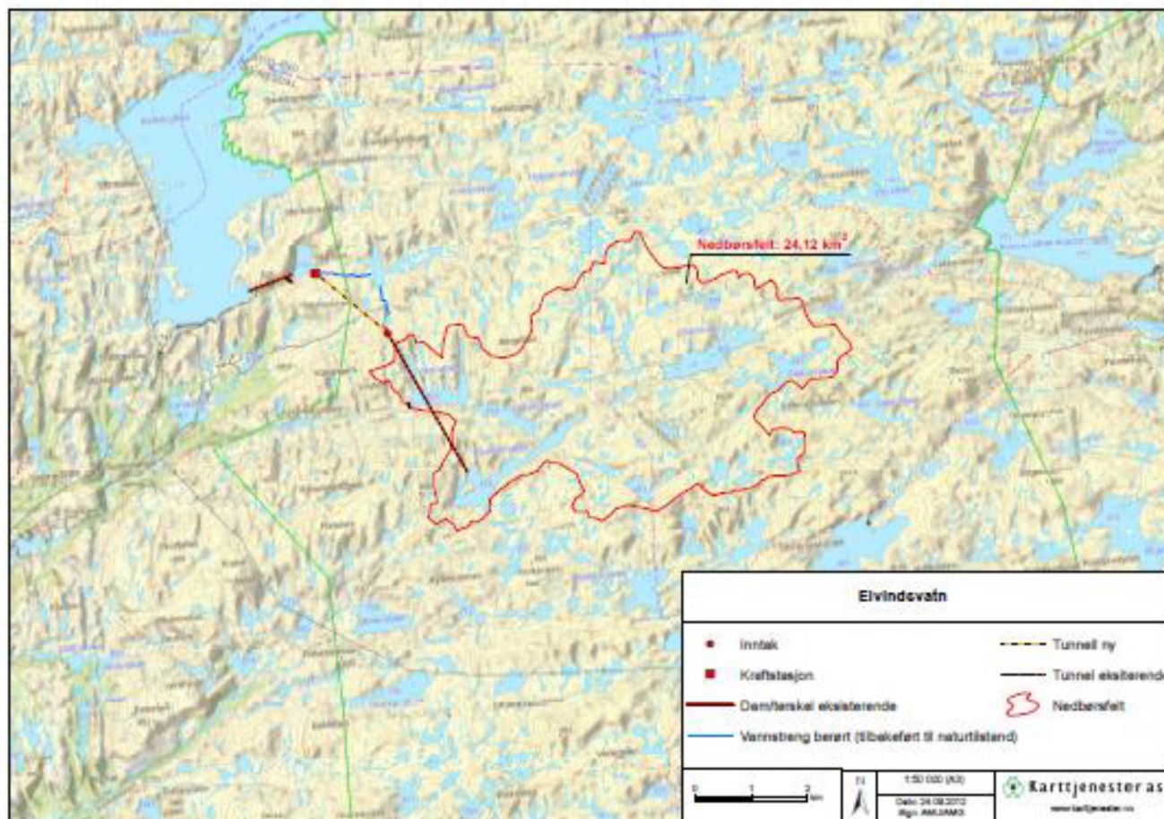
Figur 2.2 Nedbørfeltet til Eivindsvatn kraftverk (kart i A4-versjon i vedlegg)
