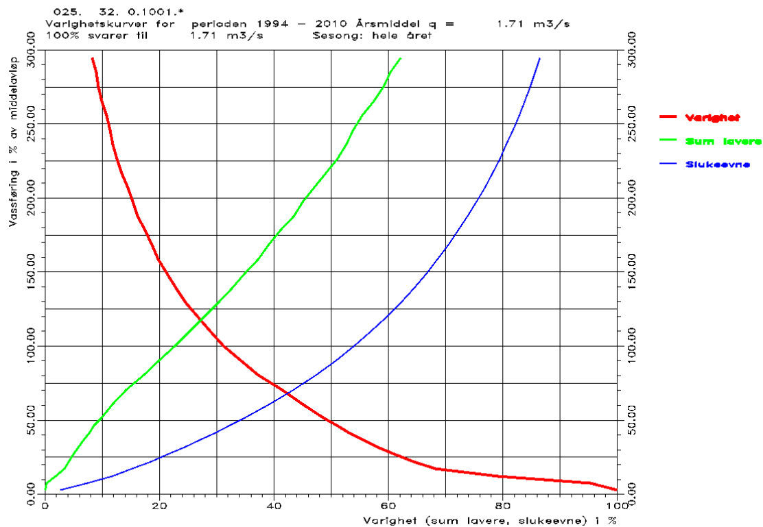
FIGUR 15: VARIGHETSKURVE, KURVE FOR FLOMTAPP OG FOR TAPP AV VANN I LAVVANNSPERIODEN (ÅR).
