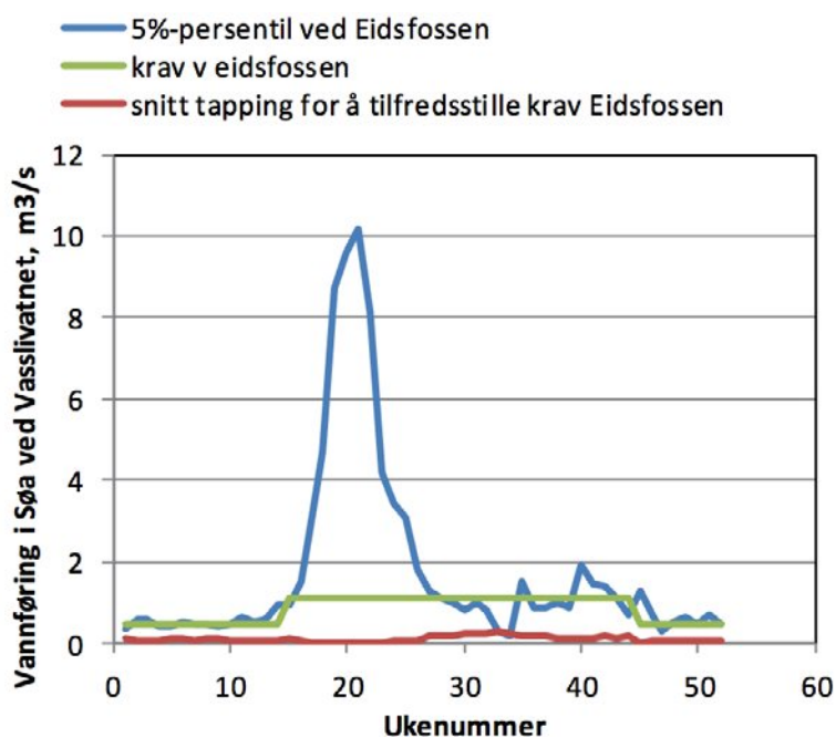
Figur 44: Fordeling over året av 5%-persentil av uregulert vannføring i Sòa ved Vasslivatnet, sammen med en naturlig sesongvariasjon av minstevannslipp (sommer fra og med uke 15 til og med uke 44)
