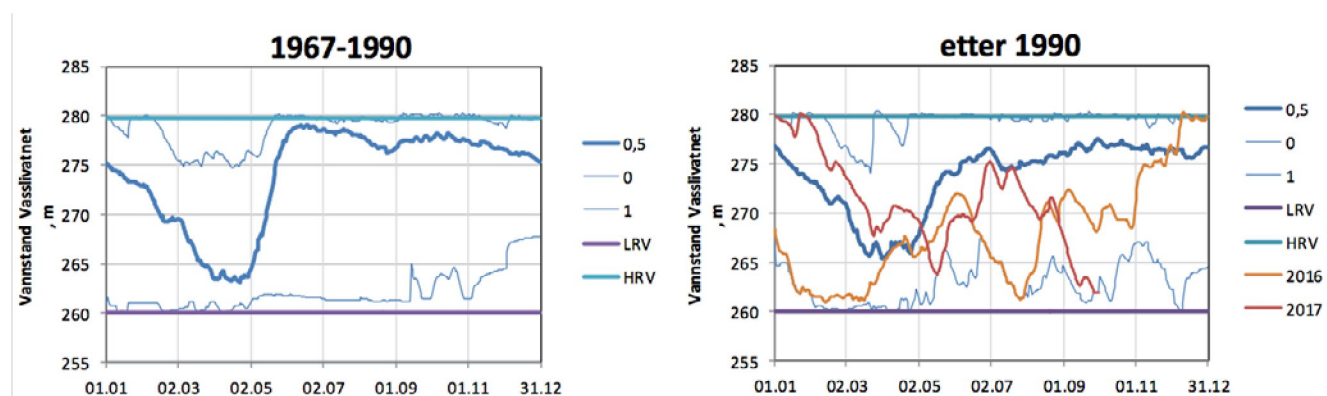
Figur 24 : Vannstandsvariasjon gjennom året for Vasslivatnet. . Kurvene merket 0.5, 0 og 1 er hhv 50%- 0%- og 100%-persentilene til vannstanden i de kalenderårene som er angitt i figuren.
