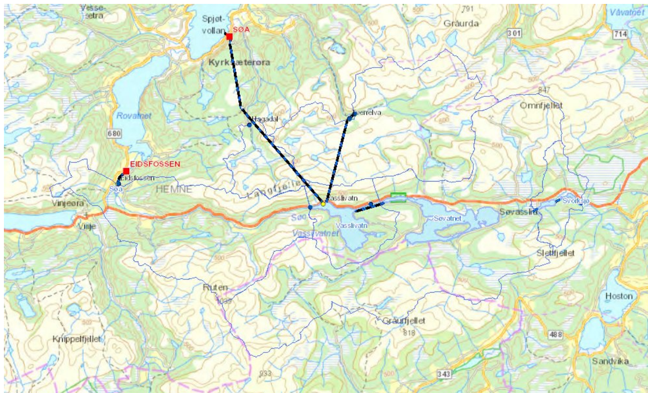
Figur 2 : Oversiktskart over Sør-reguleringen med nedbørsfelt, magasiner, kraftverk og tunneler.
