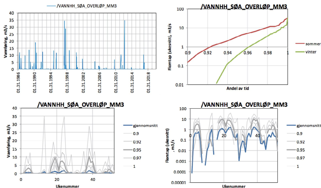
Figur 18 : Statistikk for flomtap fra Sør kraftverk, fra ukentlig vannhusholdning fra 1986-2016
