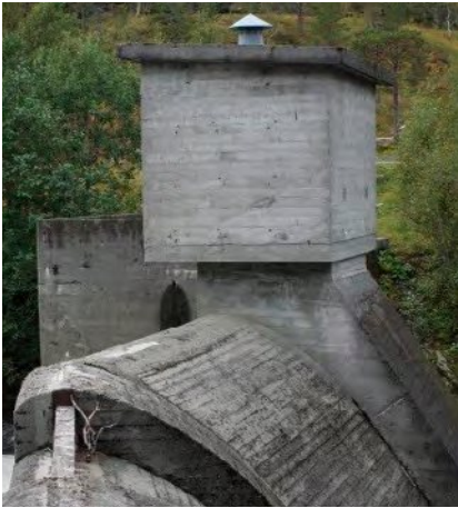
Figur 12 : Inntak Hagaelva.
