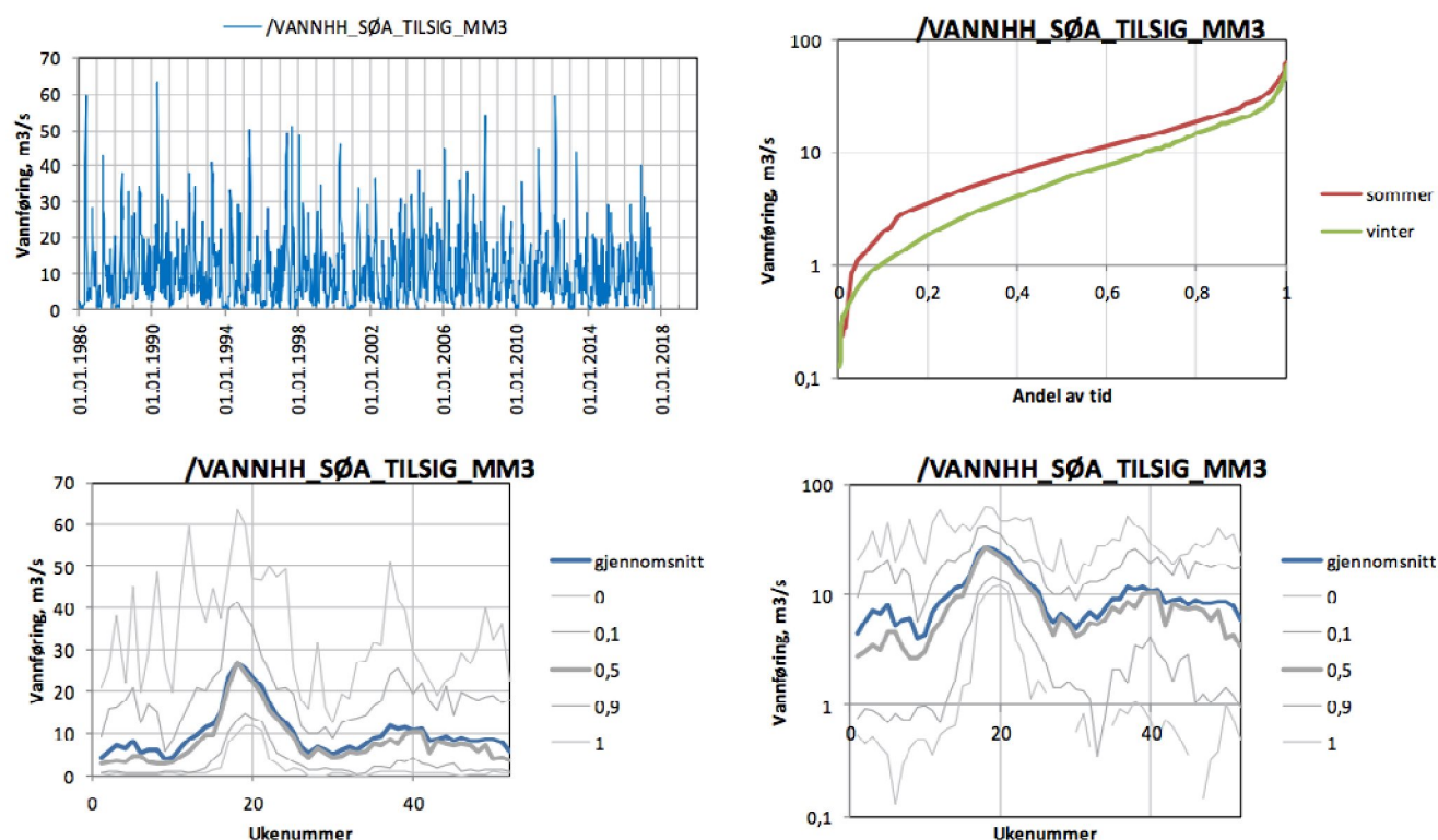
Figur 17 : Statistikk for tilsiget til hele Sør kraftverk, inkludert overføringer.
