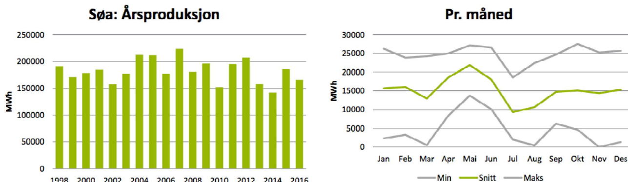
Figur 37 : Produksjonsstatistikk vist år for år og fordelt pr. måned
