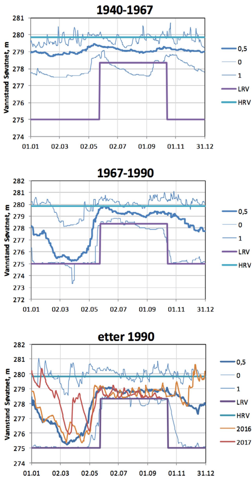
Figur 22 : Variasjon av vannstand gjennom året, for Søvatnet. Kurvene merket 0,5, 0 og 1 er hhv 50%- 0%- og 100%-persentilene til vannstanden i de kalenderårene som er angitt i figuren.
