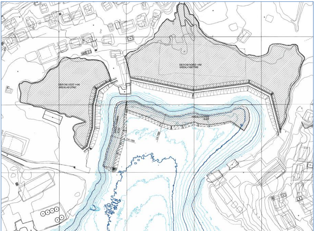
Foreløpig prosjekterte fyllinger, Kystverket
