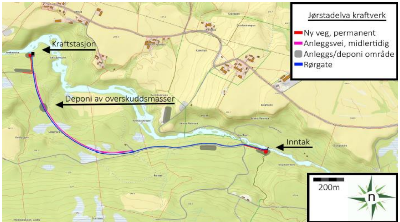
Figur 2: Detaljkart Jørstadelva kraftverk.
