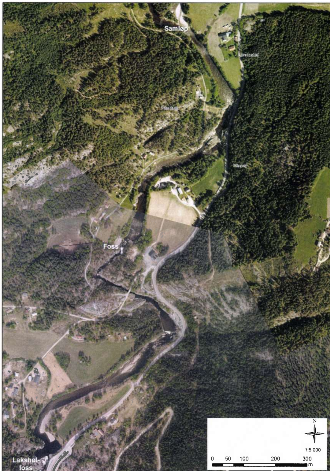
Satellittbildet viser Vallaråi fra Lakshølfoss og opp til samløpet med Grunnåi, til sammen en elvestrekning på 2 km. Mulig vandringshindrende foss i øvre del av Satajuvet er markert.
