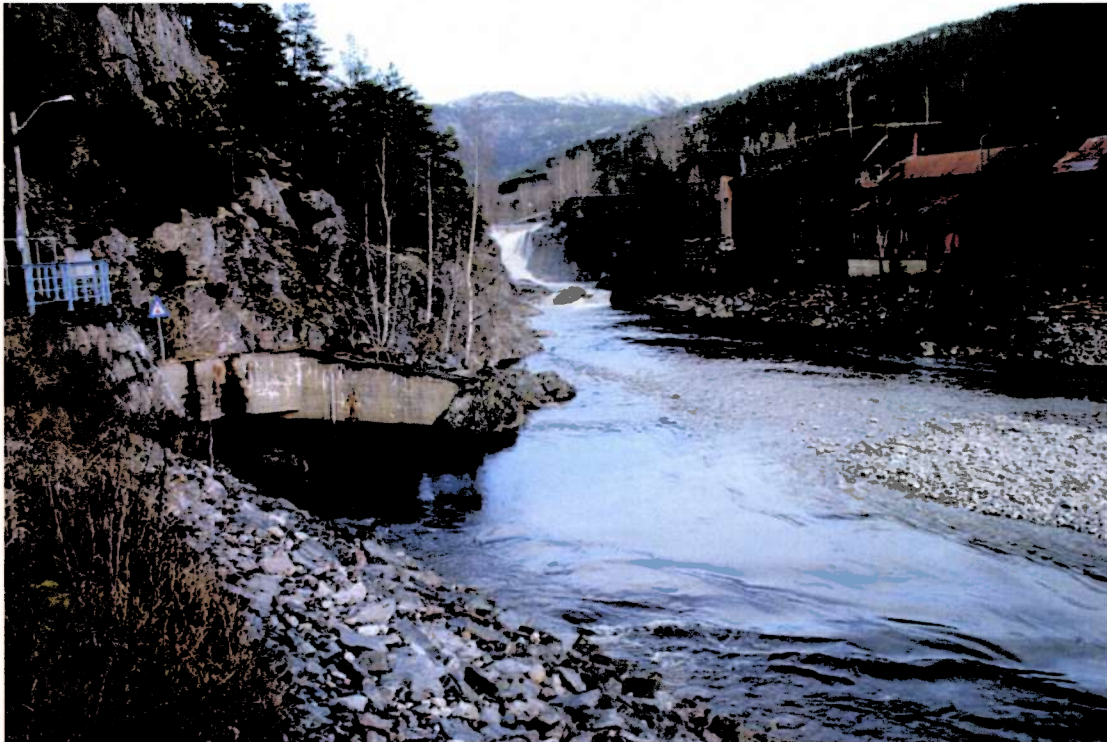
Figur 1. Driftsvannet fra Sundsbarm kraftverk møter vannføringen fra øvre del av Vallaråi fra Flatdal. Lakshølfoss og Laksehøl sees oppstrøms samløpet.
