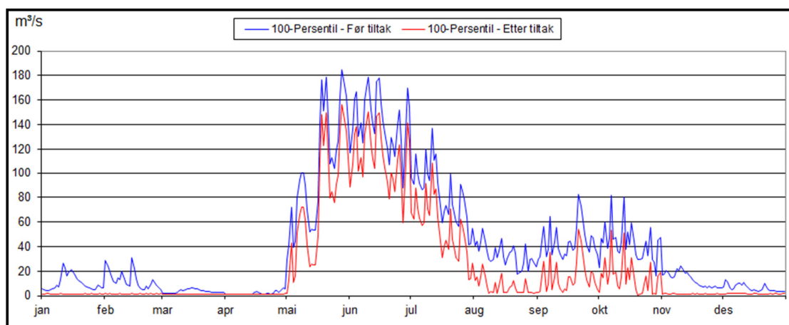
Vedlegg 2 - Figur 2 Vannføringen i Ranaelva, ved beregningspunkt 2 (1967-2011), daglige verdier før og etter utbygging. Minimumsvannføringer (0-persentil) øverst, medianvannføringer i midten og maksimumsvannføringer (100-persentil) nederst.
