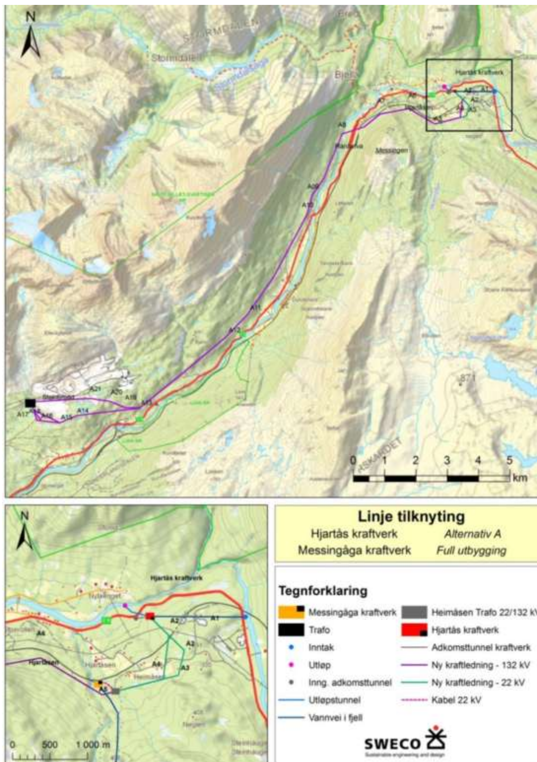
Figur 3-4 Planlagt kraftledning mellom Hjørtås kraftverk og Ørtfjellmoen transformatorstasjon. Utbygging etter alternativ A er vist.
