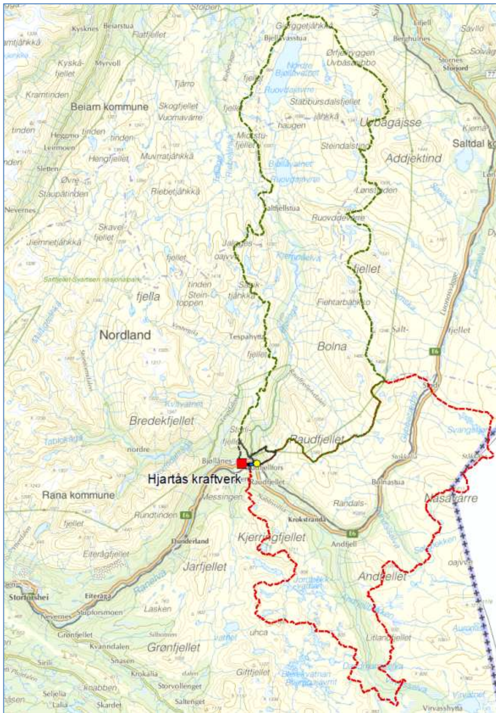
Figur 5-1 Tilsigsfelt (stiplet rødt), restfelt (stiplet grønt/grått) for Hjørtås kraftverk
