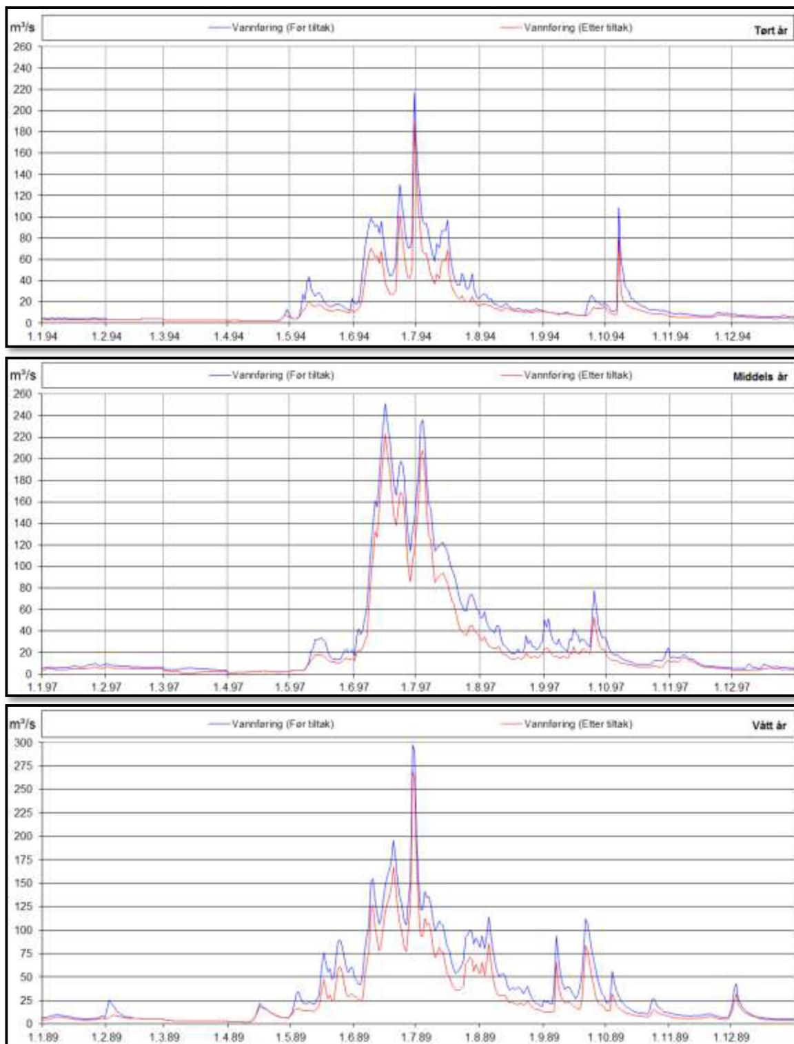
Figur 5-7. Beregnet vannføring før og etter utbygging, rett nedstrøms samløp med Bjellåga, i et tørt år (1994), et "middels" år (1997) og et vått år (1989). Kilde: Sandsbråten 2013.
