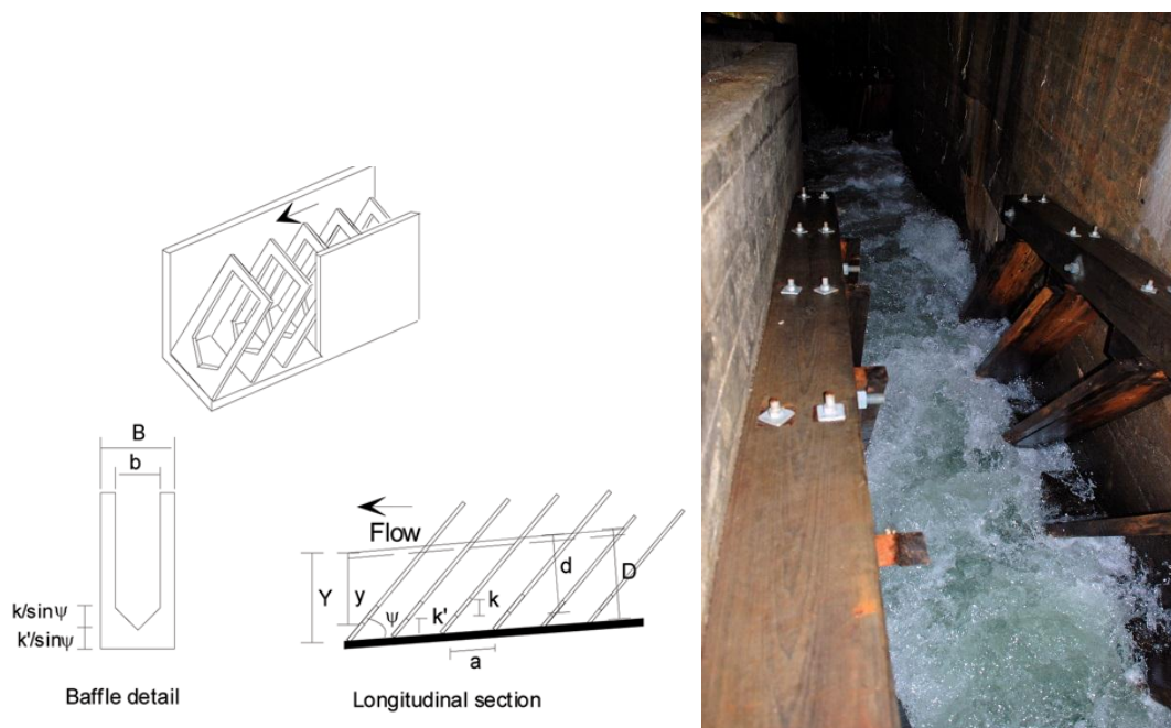
Figur 6. a Oppbygging av motstrømstrapper. Figur etter Katopodis 1992. b. Motstrømstrapp i dammen ved Hunderfossen kraftverk. Foto: Morten Kraabøl, NINA.
