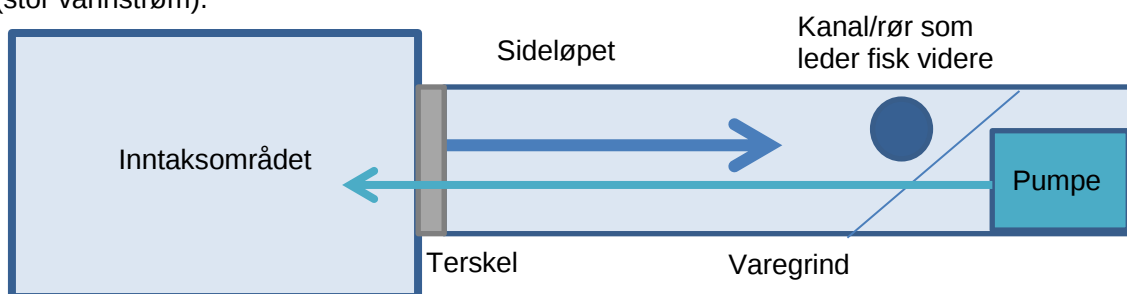
Figur 2. Skisse over prinsipløsning (sett ovenfra) for å pumpe vann tilbake til produksjon.
