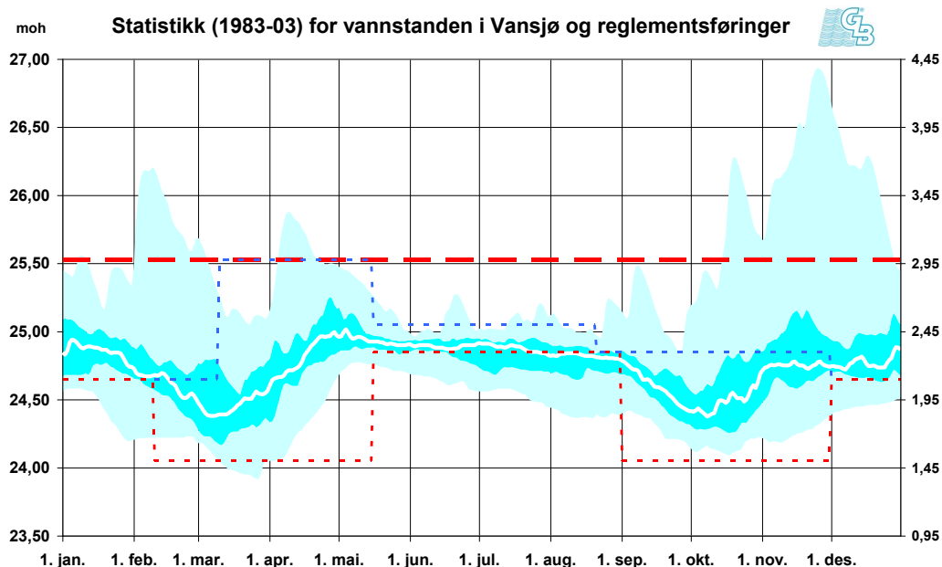
Figur 2. Reglementsføringer for vannstanden i Vansjø og statistikk for perioden 1983-2003. Figuren er utarbeidet av GLB.
