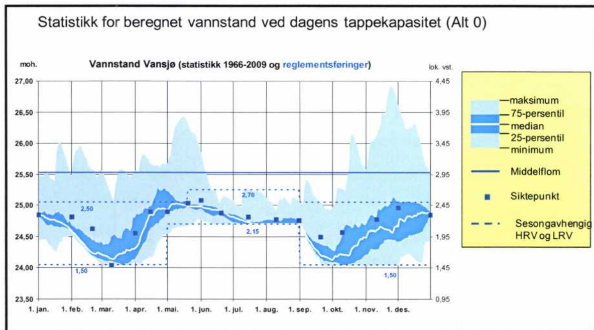
Figur 6.4. Statistikk for simulert vannstand i Vansjø i perioden 1966-2009 ved dagens tappekapasitet. Vannstanden søkes å ligge innenfor sesongavhengig høyeste og laveste regulerede vannstand i prøvereglementet.
