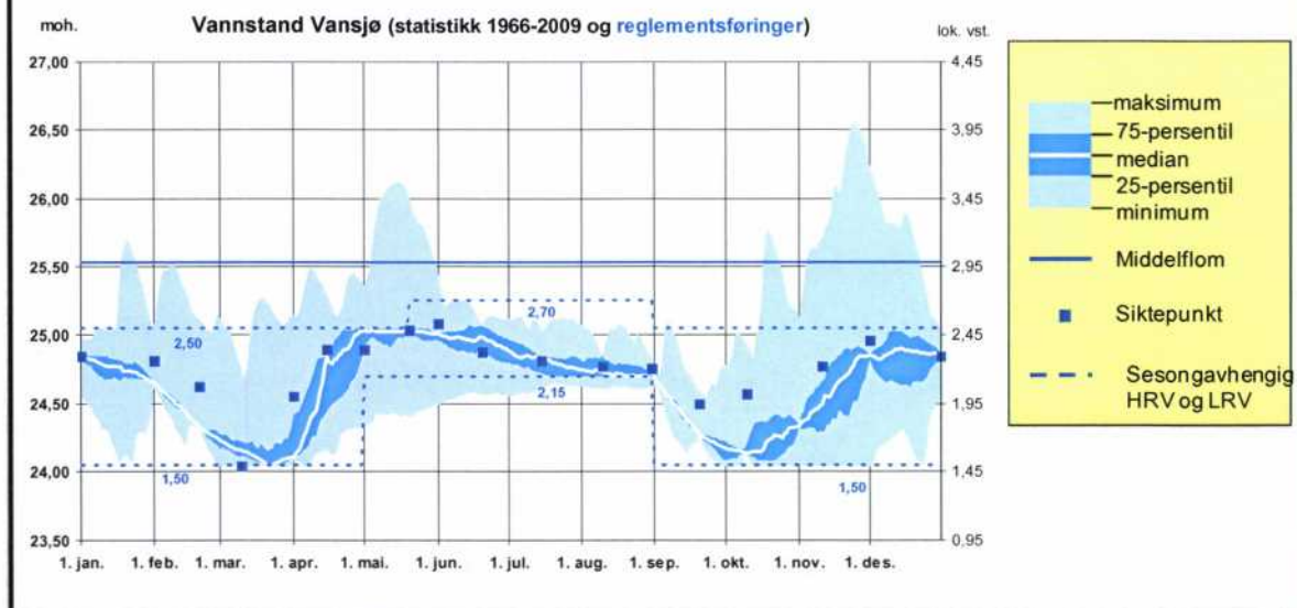
Figur A3. Statistikk for beregnet vannstand i Vansjø i årene 1966-2009 for alternativ II+A.
