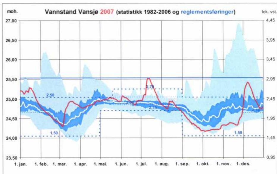
Figur 3.3. Glommen og Lågens Brukseierforenings oversikt over vannstanden i Vansjø sommeren 2007, sett i relasjon til normalvannstand 1982-2006 (hvit linje), samt reglementsføringer (mørk blå linjer).
