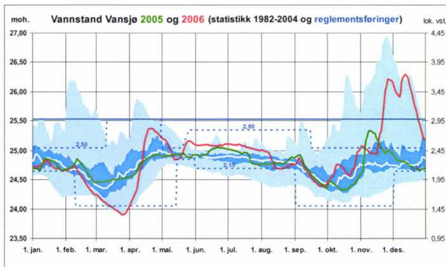
Figur 3.1. Sommertappinger i 2005 (grønn linje) og 2006 (rød linje).
