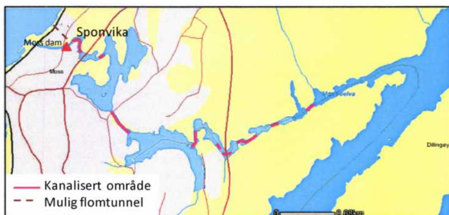
Figur 6.2. Kart over kanaliserte områder i beregningene. Parsellen i Sponvika er betegnet som Nedre del, og er i dag svært trang, med tilhørende stort falltap. De åtte øvrige parsellene utgjør Øvre del. Mulig flomtunnel fra Moss dam til Mossefjorden er også vist. Utsnittets beliggenhet er vist i figur 6.1.
