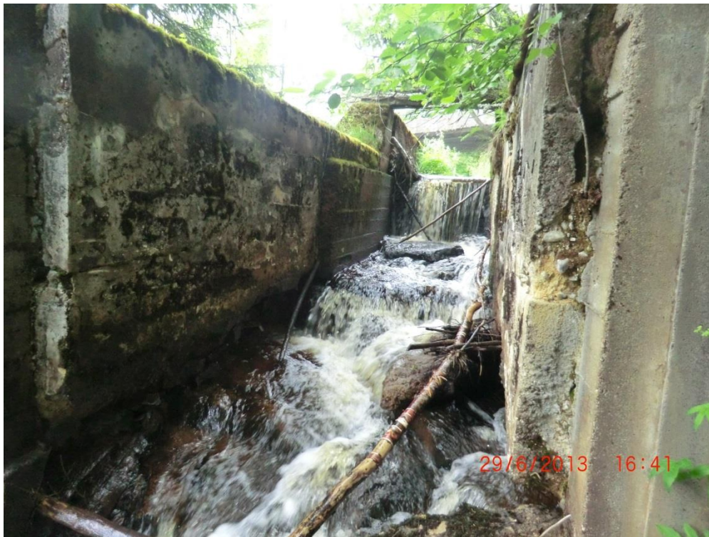
Bilde 3: Gammel inntakskanal. Her kommer også ny inntakskanal
