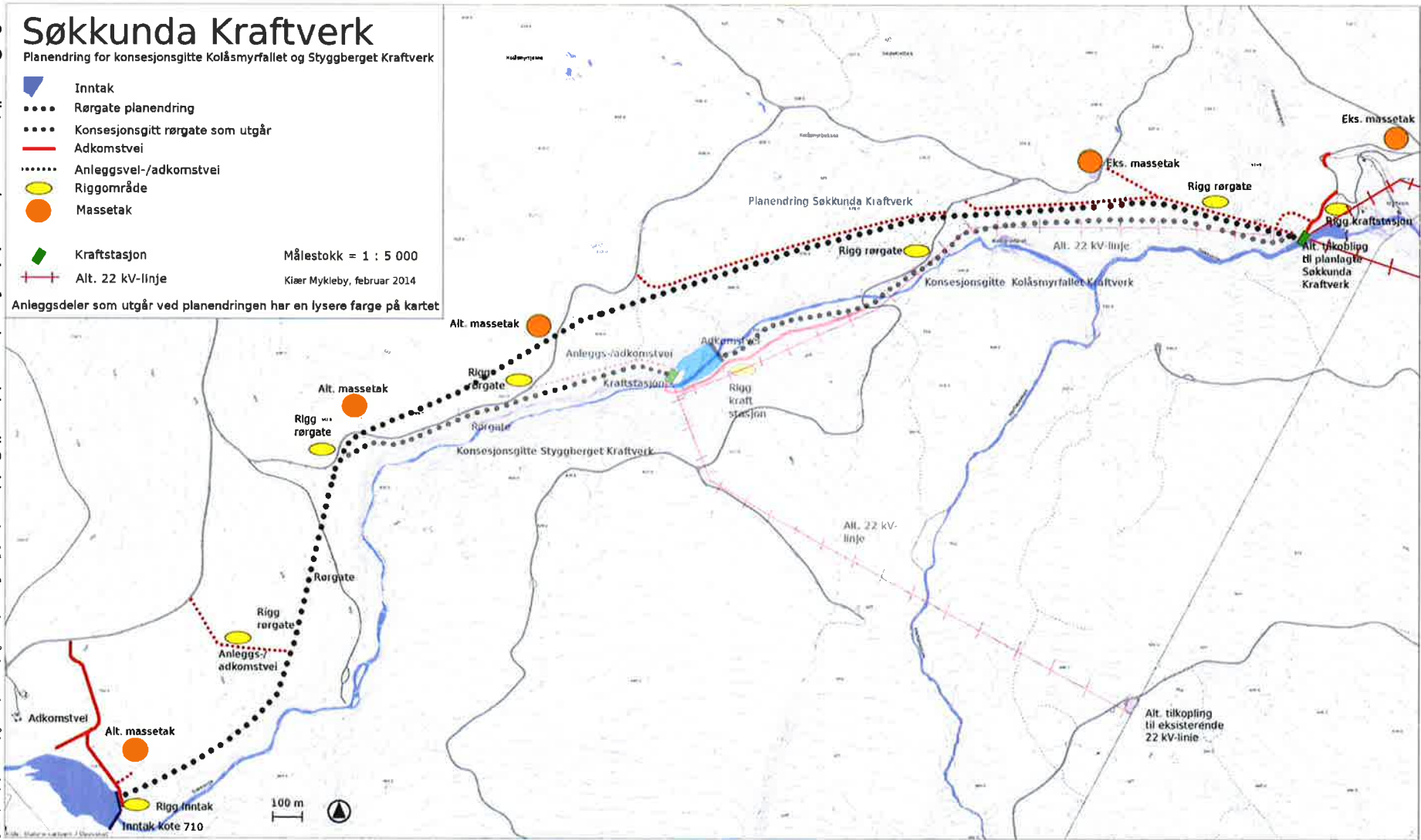
Figur 2: Oversikt over anleggsdeler for planending til Søkkunda Kraftverk på kart i målestokk 1:5000.
