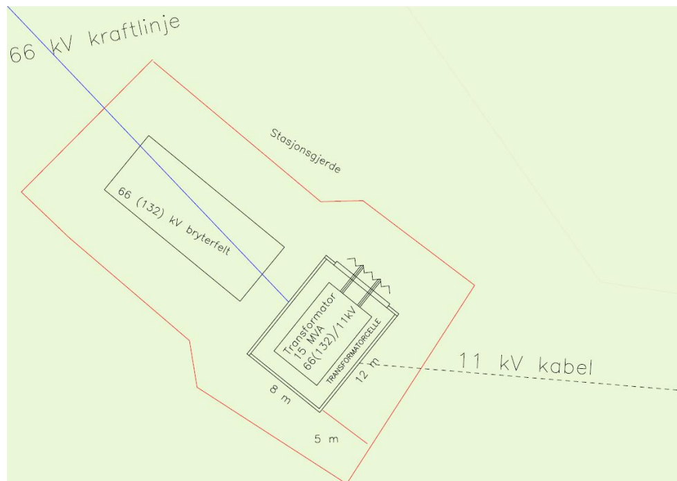
Figur 2-5 Planskisse transformator og koblingsanlegg.
