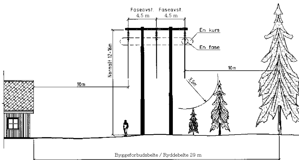
Figur 2-7 Masteskisse av H – mast for 132 kV ledning med byggeforbudsbelte 29 m, skissen er hentet fra vedlegg 13.
