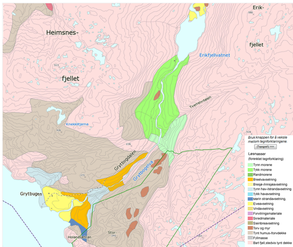
Figur 2-1 Løsmassekart Grytbogelva og Tverrelva.
