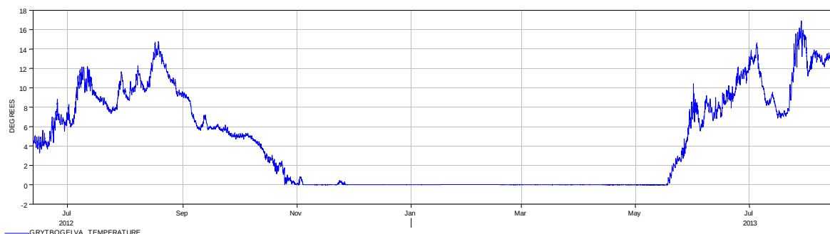
Figur 3-7 Vanntemperatur i Erikfjellvatnet på 1 meters dyp.
