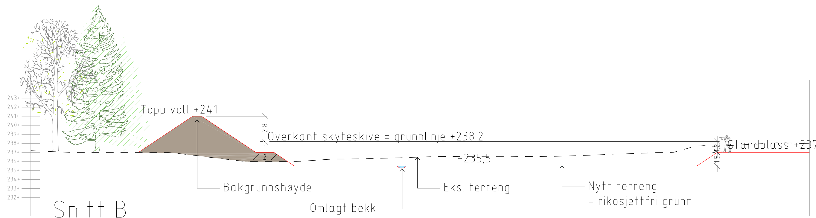
Snitt / oppriss C
