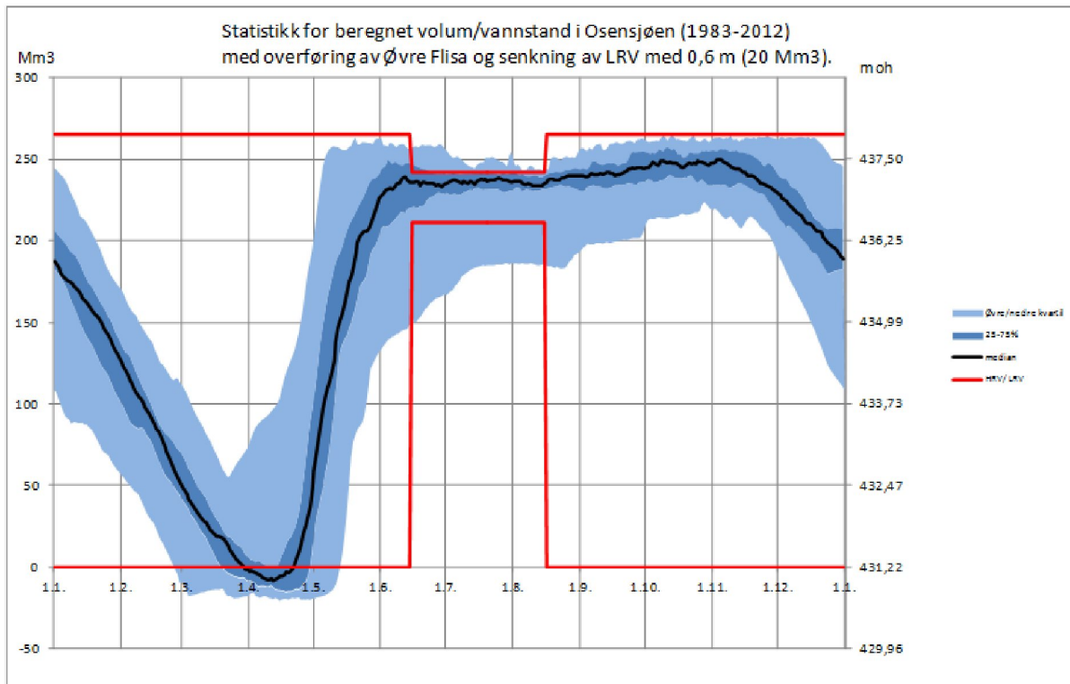
A2. Statistikk for beregnet volum/vannstand for Osensjøen (1983-2012) med overføring av Øvre Flisa og senkning av LRV med 0,6 m (20 Mm 3 ). Figuren illustrerer også alternativ AB2 (overføring av Øvre Flisa og Østre-Æra).
