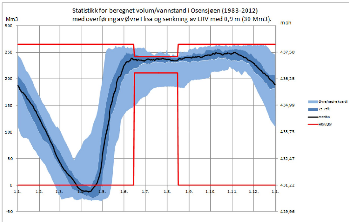
A3. Statistikk for beregnet volum/vannstand for Osensjøen (1983-2012) med overføring av Øvre Flisa og senkning av LRV med 0,9 m (30 Mm 3 ). Figuren illustrerer også alternativ AB3 (overføring av Øvre Flisa og Østre Æra).
