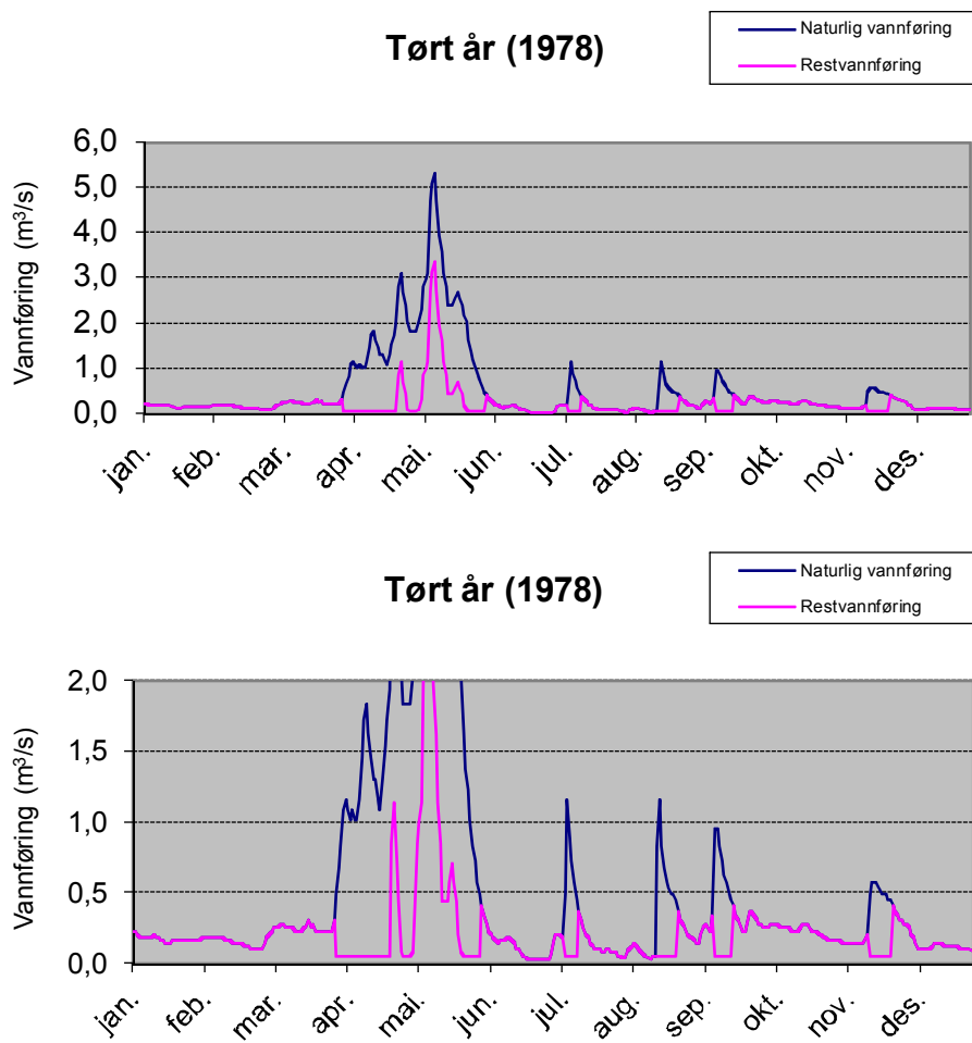
Figur 6. Plott som viser vannføringsvariasjoner i et tørt (1978) år (før og etter utbygging). 17
