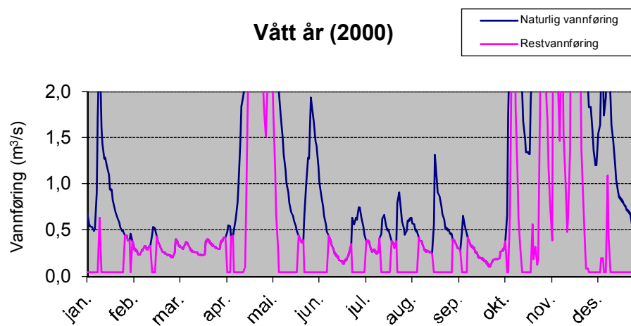
Figur 8. Plott som viser vannføringsvariasjoner i et vått (2000) år (før og etter utbygging). 19
