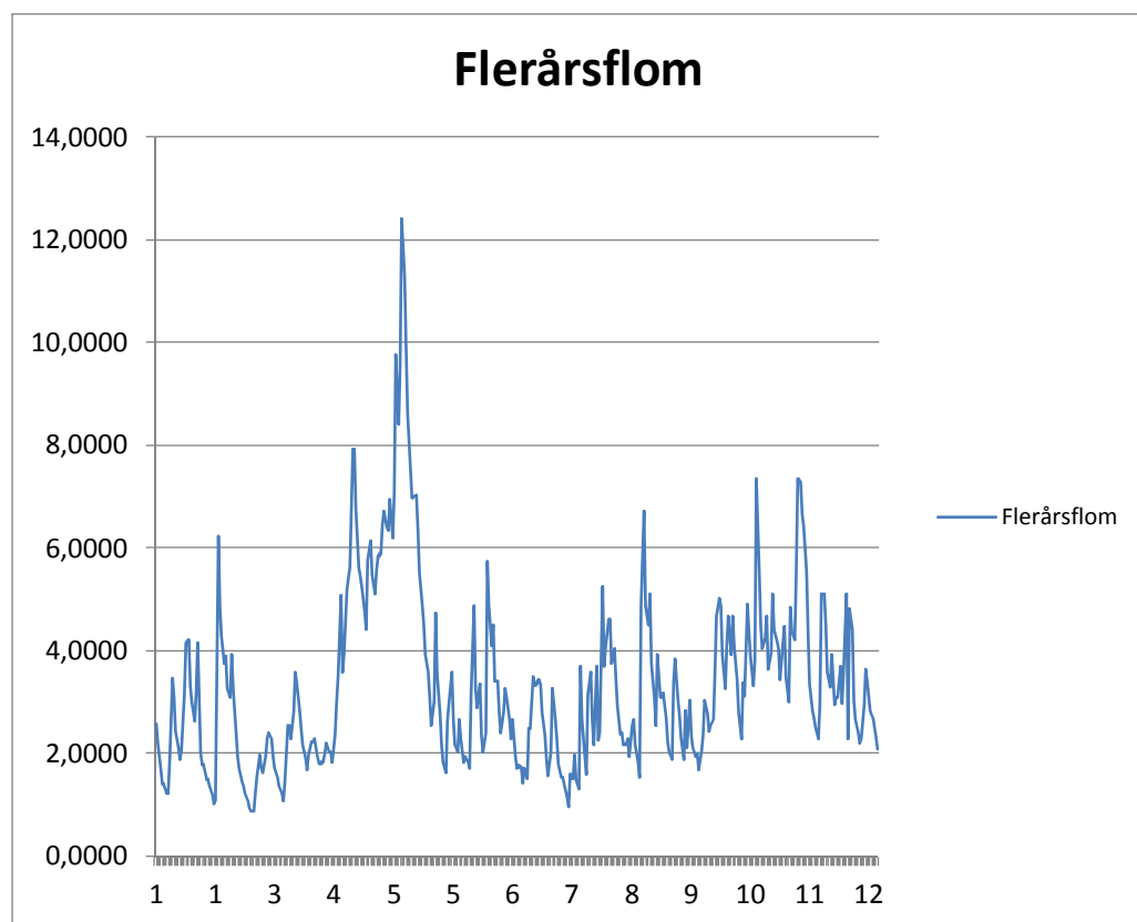
Figur 4. Plott som viser sesongvariasjon i maksimumsvannføringer gjennom året (døgndata). 15
