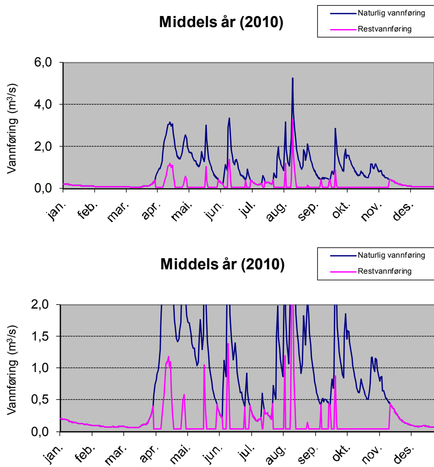
Figur 7. Plott som viser vannføringsvariasjoner i et middels (2010) år (før og etter utbygging). 18
