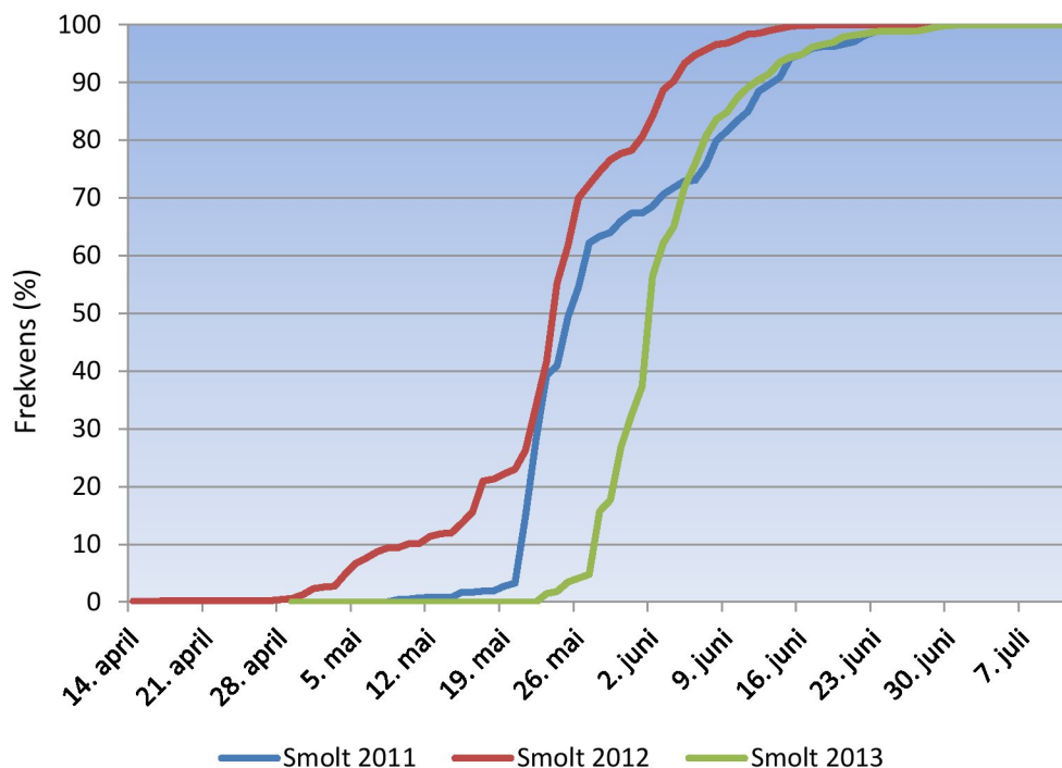
Figur 12. Kumulativ utvandring av smolt (laksesmolt og sjørretsmolt samlet) registrert med et undervannsvideosystem på dam Mannflåvann i årene 2011 til 2013.
