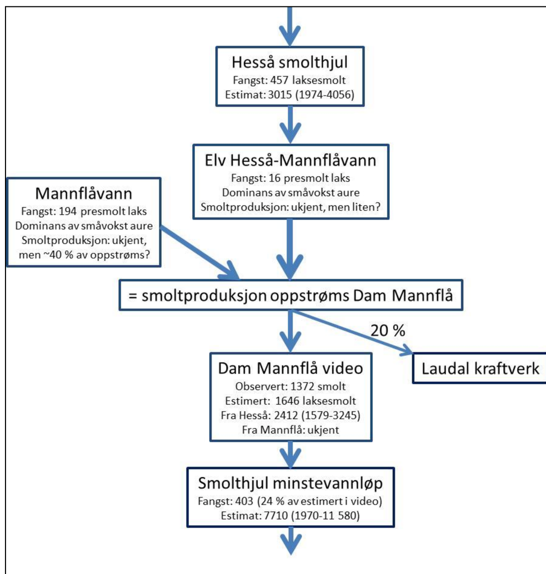
Figur 14. Prinsippsskisse som viser smoltmengdene i ulike deler av Mandalselva oppstrøms minstevannstrekningen ved Laudal basert på undersøkelsesprogrammet våren 2013.
