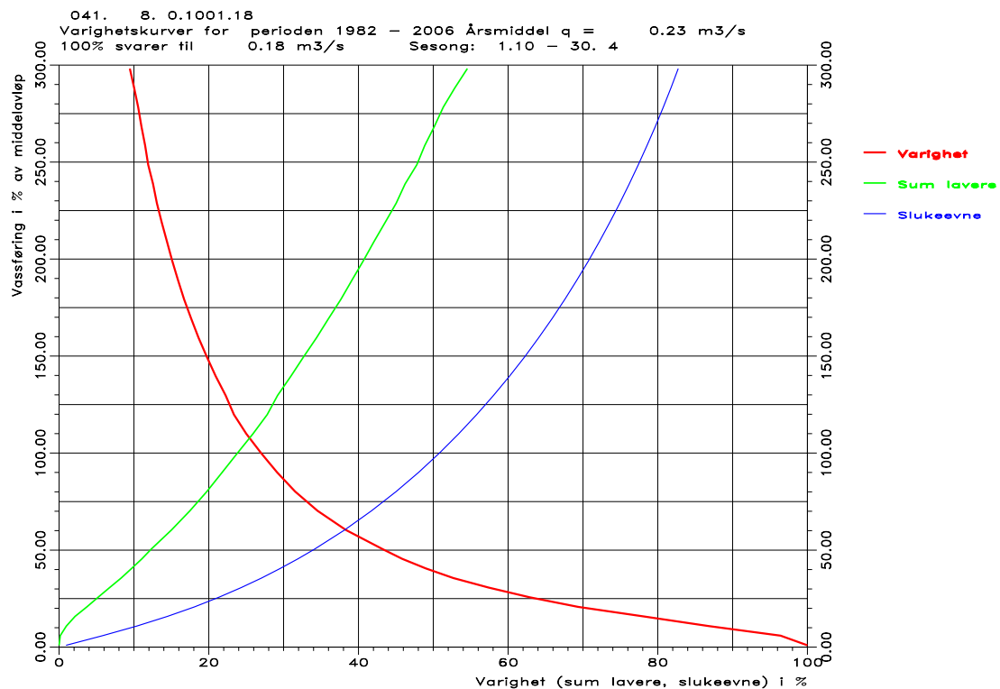
Varighetskurve, vintersesong. 01.10-30.04
