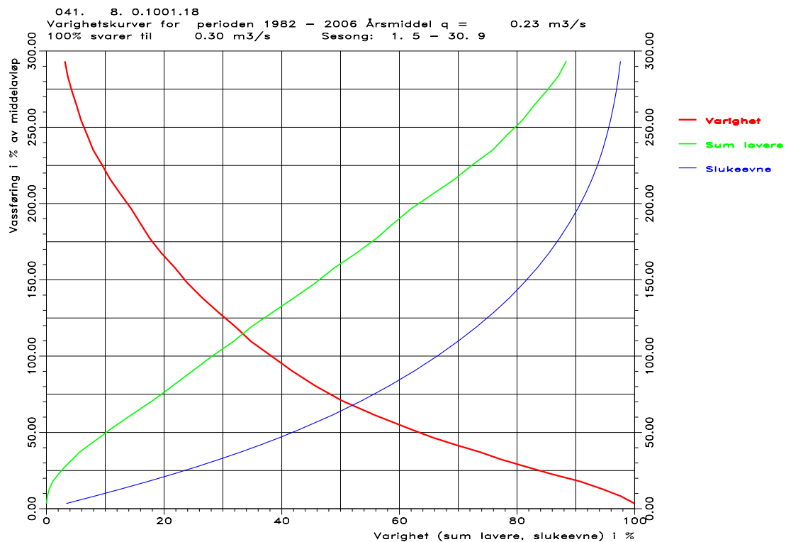
Varighetskurve, sommersesong 01.05 – 30.09
