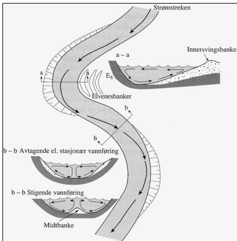
Figur 2. Strømmønsteret i elver. Pilene viser strømsbreken, linja som forbinder punktene langs elveløpet der vannhastigheten er størst. Strømsbreken forklarer hvorfor elva eroderer yttersvingene (sideerosjon) mens materiale sedimenteres som innersvingbanke i innersvingene /2/.
