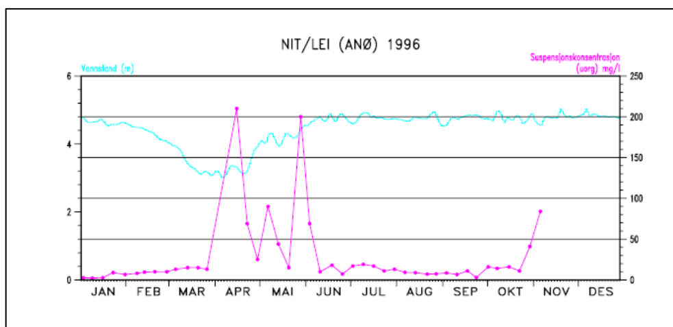
Figur 4. Oversikt over suspendert materiale (mg/l SS) og vannstand (m) i Nitelva i perioden januar – november 1996 /4/.
