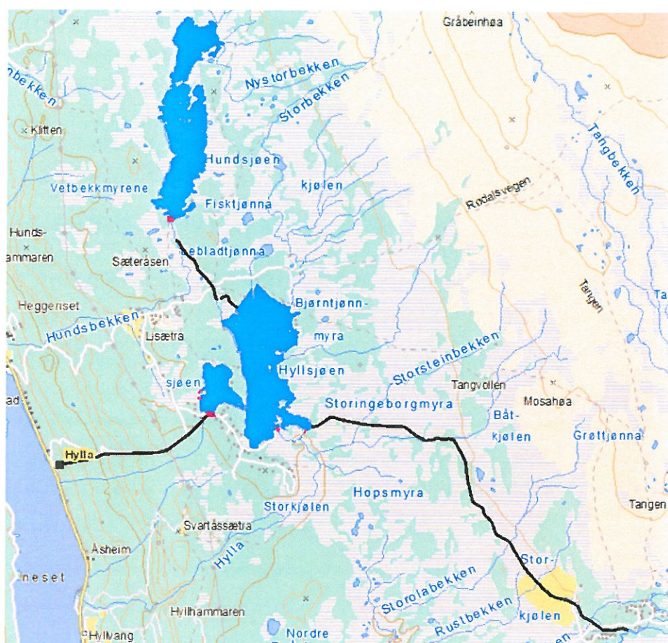
Figur 1: Kartutsnitt av Hyllsjøen, Hundsjøen, overføringen fra Hundsbekken, overføringen fra Røa, samt rørgaten fra Hyllsjøen til Hylla kraftverk (NVE Atlas).
