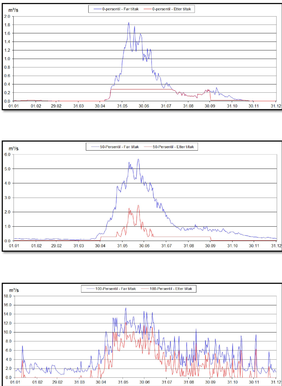
Figur 28 Vannføringen i Silåga, ved beregningspunkt 2 (1973-2013), daglige verdier før og etter utbygging. Minimumsvannføringer (0-persentil) øverst, medianvannføringer i midten og maksimumsvannføringer (100-persentil) nederst.
