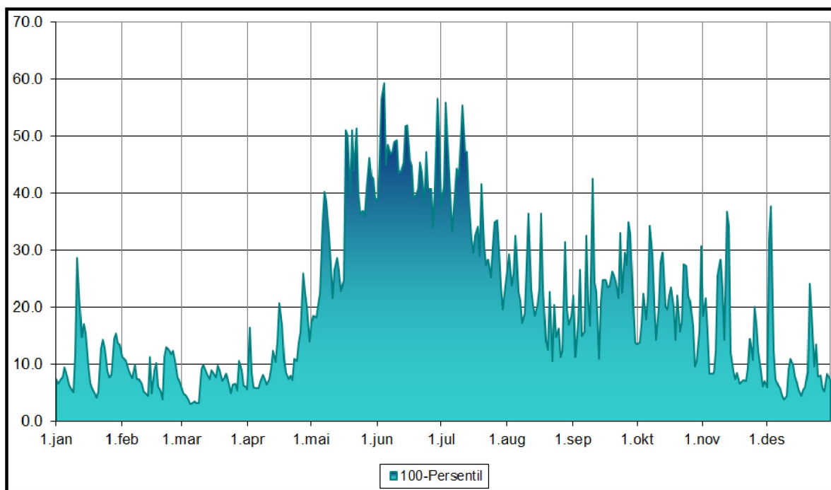
Figur 11 Daglig maksimalvannføring i løpet av dataperioden. Verdier i \text{m}^3/\text{s} .
