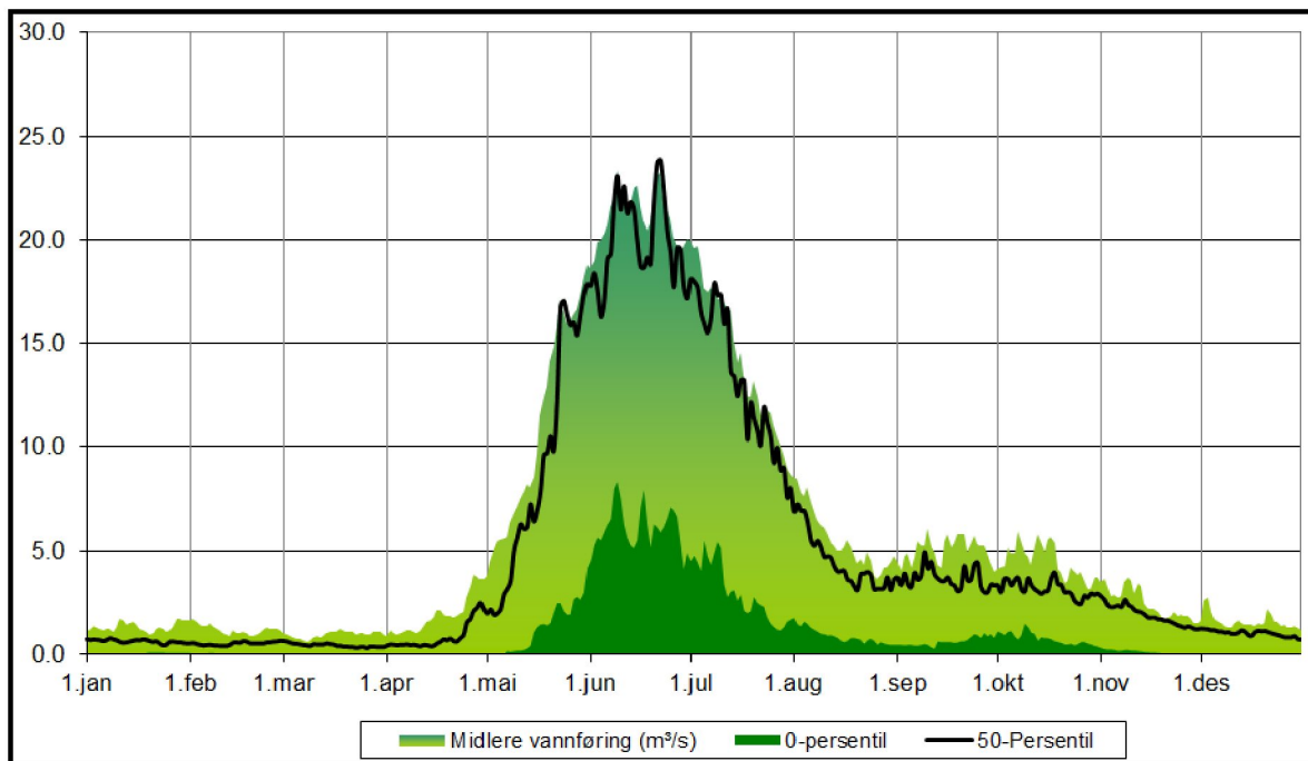
Figur 10 Midlere/median og minimumsvannføringer over dataperioden. Verdier i \text{m}^3/\text{s} .
