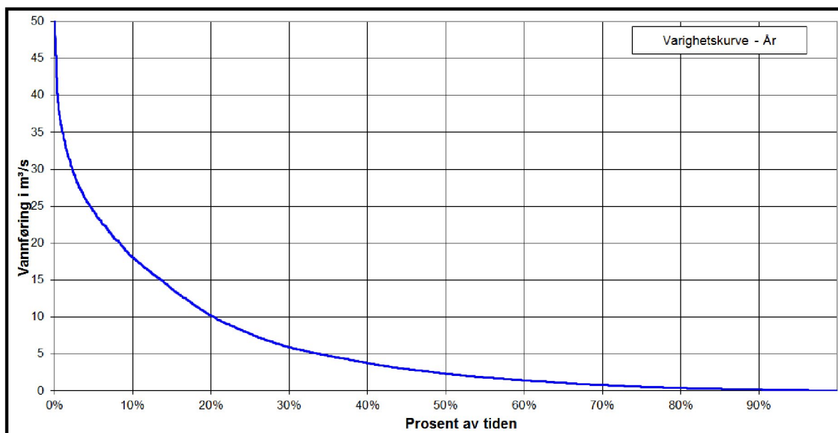
Figur 20 Varighet av vannføringer i prosent av tiden (verdier i m³/s)
