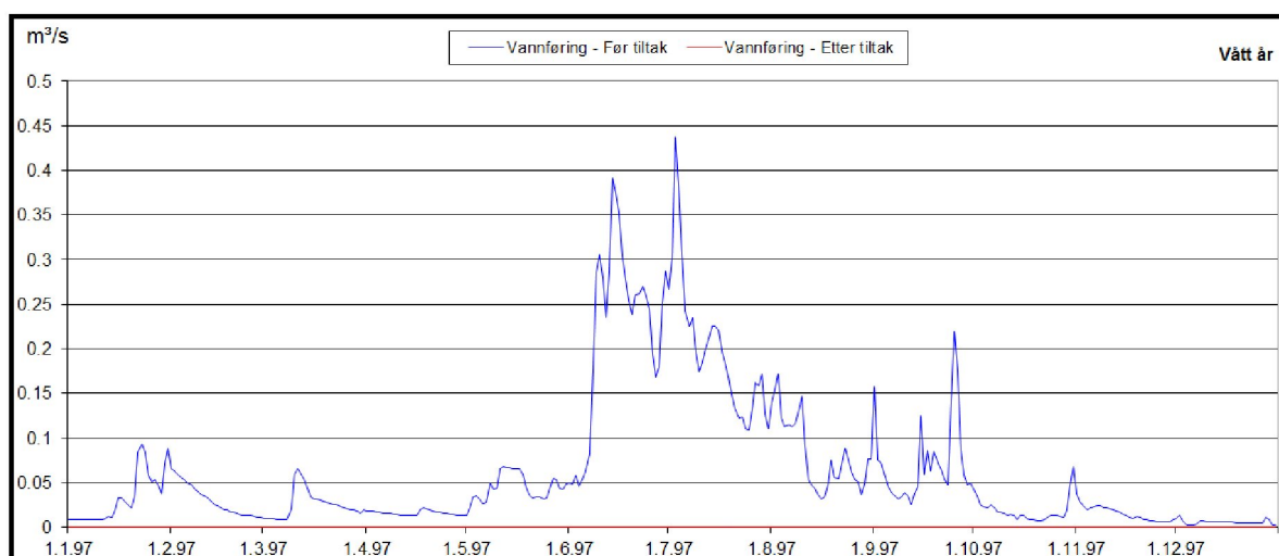
Figur 33 Beregnet vannføring før og etter utbygging, rett oppstrøms utløp, i et tørt år (1980), et "middels" år (2004) og et vått år (1997).
