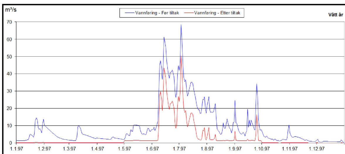
Figur 37 Beregnet vannføring før og etter utbygging, ved beregningspunkt 4, i et tørt år (1980), et "middels" år (2004) og et vått år (1997).
