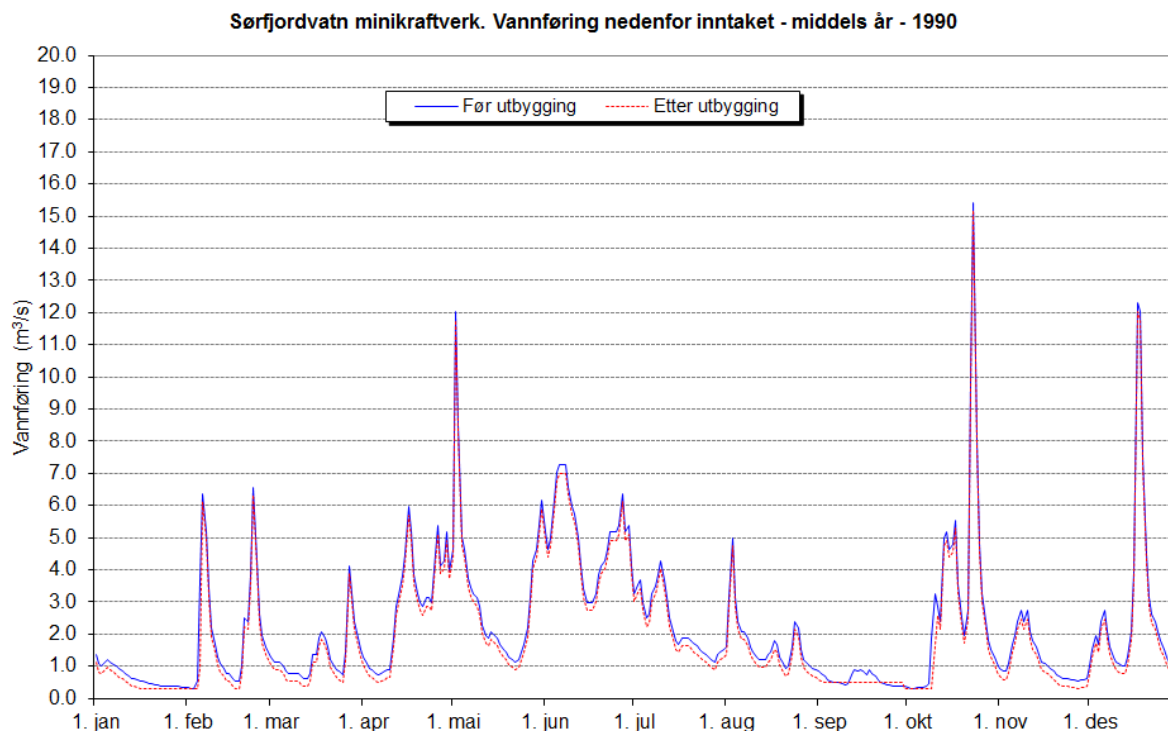
Figur 27. Plott som viser vannføringsvariasjoner i et middels (1990) år (før og etter utbygging). iv
