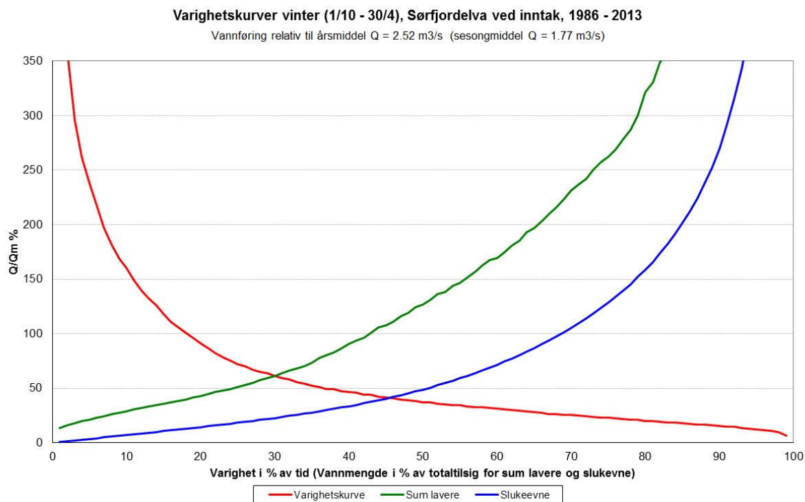
Figur 19. Varighetskurve for vintersesongen (1/10 – 30/4).
