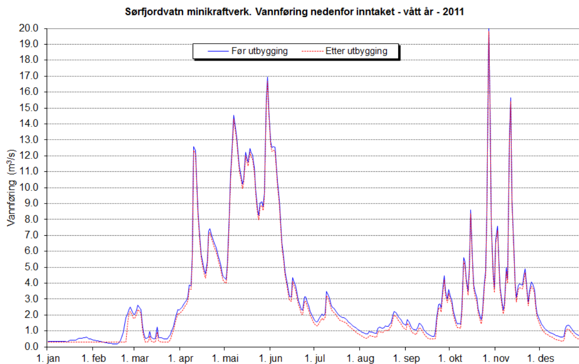
Figur 29. Plott som viser vannføringsvariasjoner i et vått (2011) år (før og etter utbygging). vi
