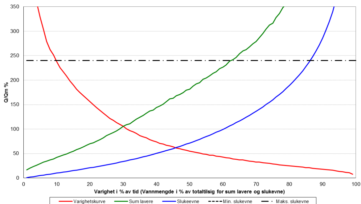
Figur 21. Varighetskurve, kurve for flomtap og for tap av vann i lavvannsperioden (år).
