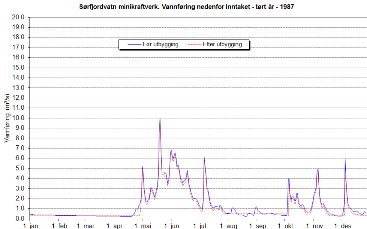
Figur 25. Plott som viser vannføringsvariasjoner i et tørt (1987) år (før og etter utbygging). ii
