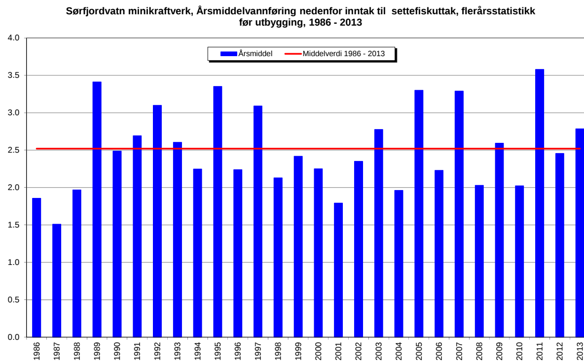
Figur 24. Plott som viser variasjoner i middelvanntføring fra år til år (år). i
