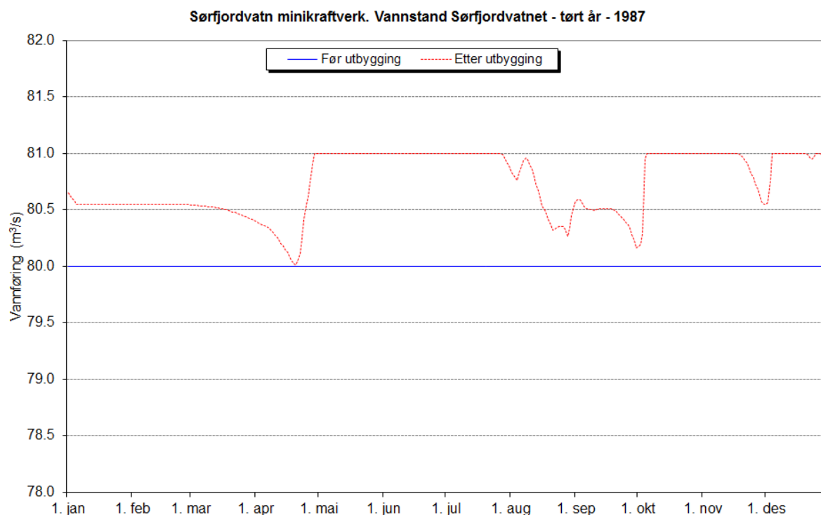
Figur 31. Vannføringsvariasjoner i Sørfjordvatnet tørt år (1987) år (før og etter utbygging)
