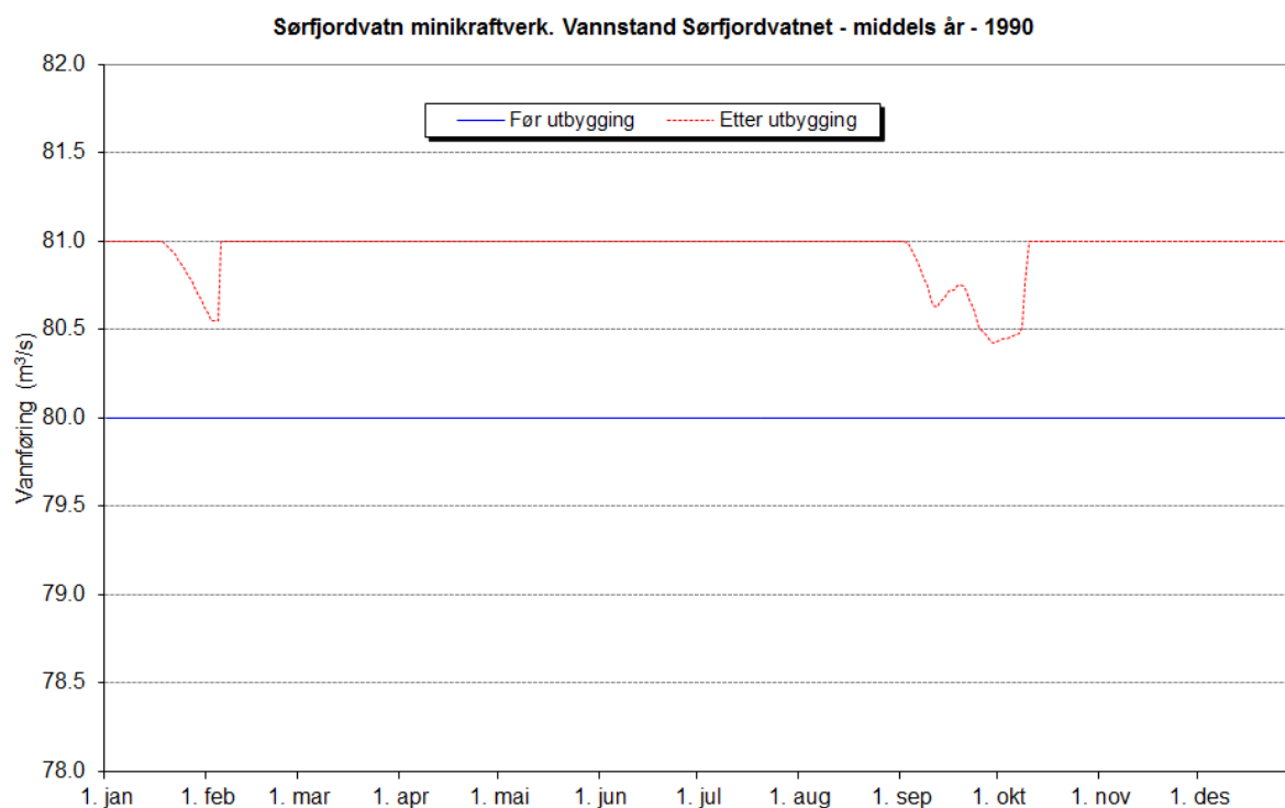
Figur 32. Vannføringsvariasjoner i Sørfjordvatnet middels år (1990) år (før og etter utbygging)
