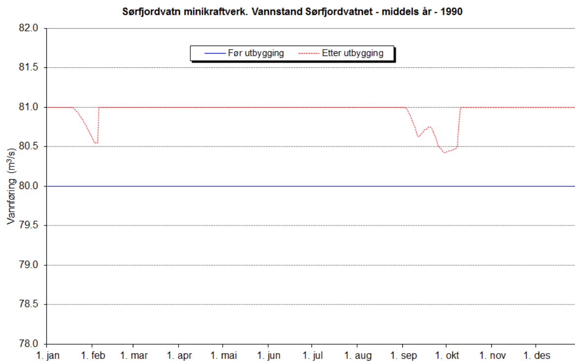
Figur 33. Vannføringsvariasjoner i Sørfjordvatnet i et vått (2011) år (før og etter utbygging)
