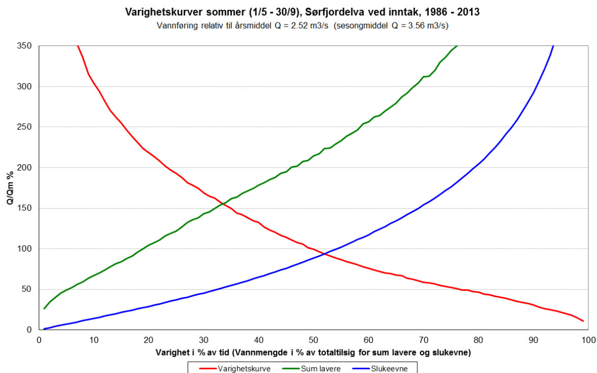
Figur18. Varighetskurve for sommersesongen (1/5 – 30/9).
