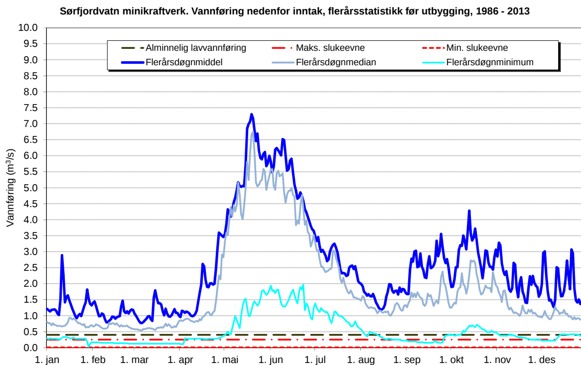
Figur 22. Plott som viser sesongvariasjon i middel/median- og minimumsvannføringer gjennom året, (døgndata). 1
