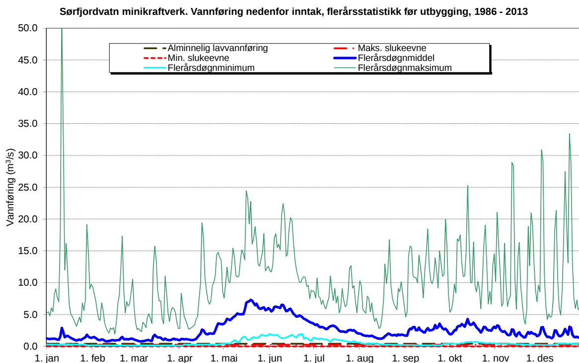
Figur 23. Plott som viser sesongvariasjon i maksimumsvannføringer gjennom året (døgndata). 2
