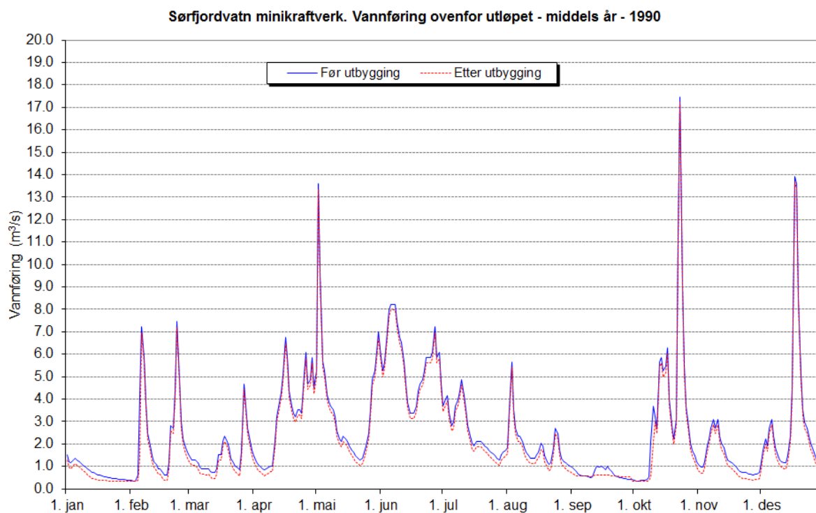
Figur 281. Plott som viser vannføringsvariasjoner i et middels (1990) år (før og etter utbygging). v
