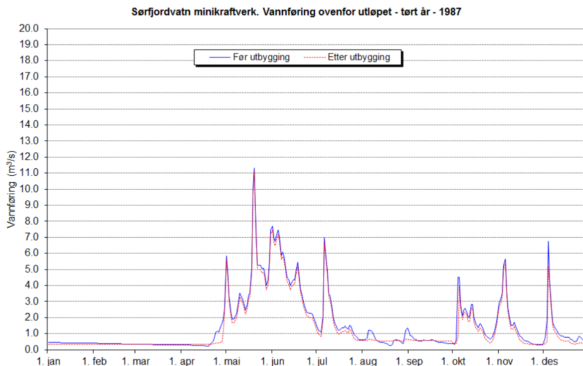
Figur 26. Plott som viser vannføringsvariasjoner i et tørt (1987) år (før og etter utbygging). iii
