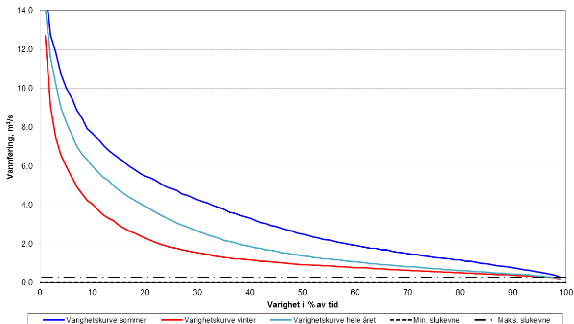
Figur 20. Varighetskurve, kurve for sommer, vinter og hele året.
