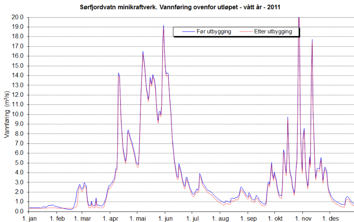
Figur 30. Plott som viser vannføringsvariasjoner i et vått (2011) år (før og etter utbygging). vii
