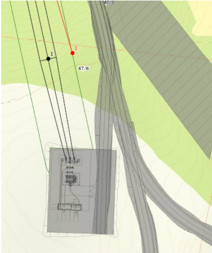
Figur 1. Rødt punkt – godkjent mastepunkt, rød strek – senterlinje godkjent trasé. Svart punkt – omsøkt mastepunkt, svart stek – faseledning omsøkt trasé.
