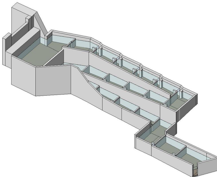
Figur 8: Skissetegning av vertikalspaltet kulpetrapp som er under oppføring ved Møllefossen. Øverst: Oversiktsbilde med inntegnet fisketrapp. Nederst: tegning av fisketrappa (kilde: Multiconsult)
