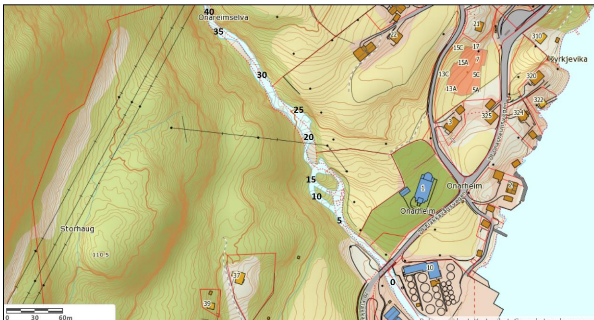
Kart over nedre delar av Onarheimsvassdraget, med høgdekotar for kvar femte meter.
