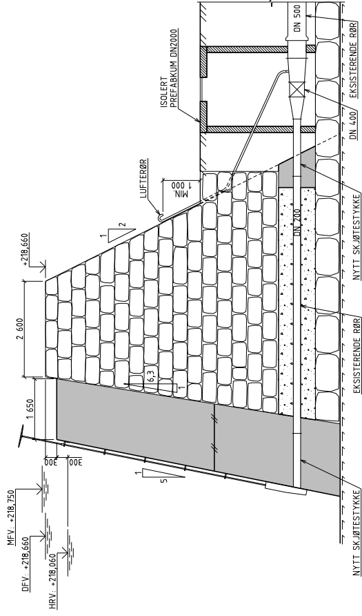
SNITT 1-1 1:50
