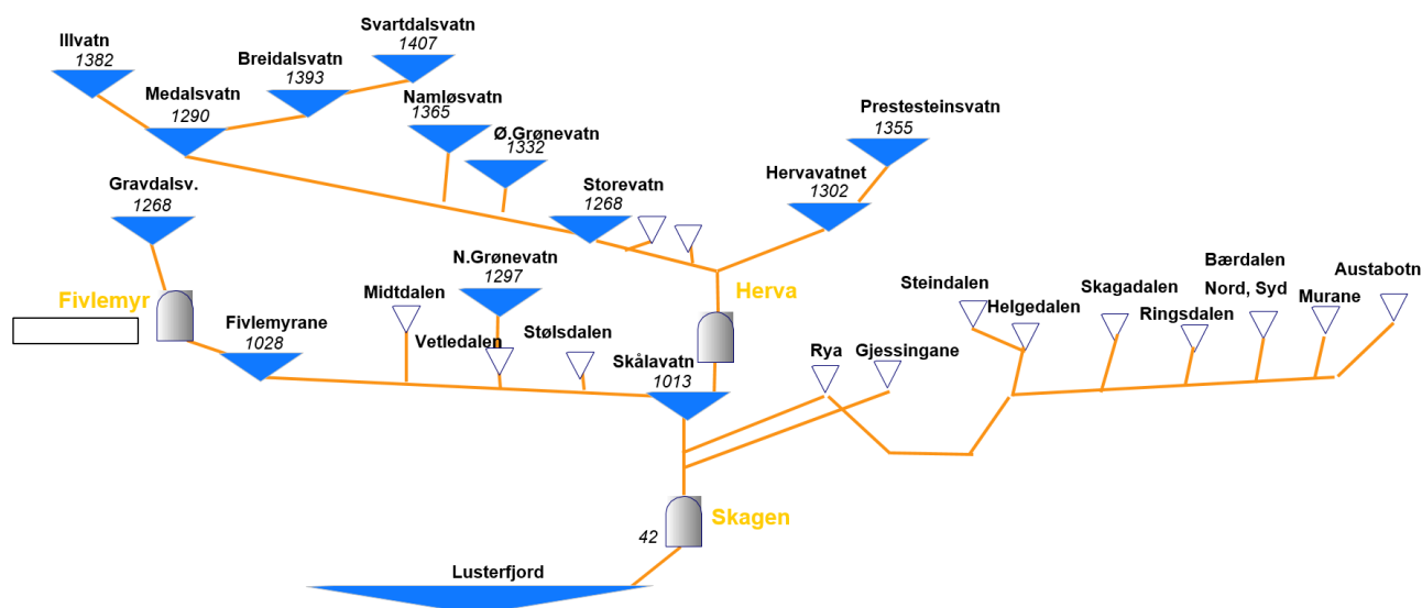
Figur 3 Hydros kraftverk og reguleringer i Fortun-Grandfasta
