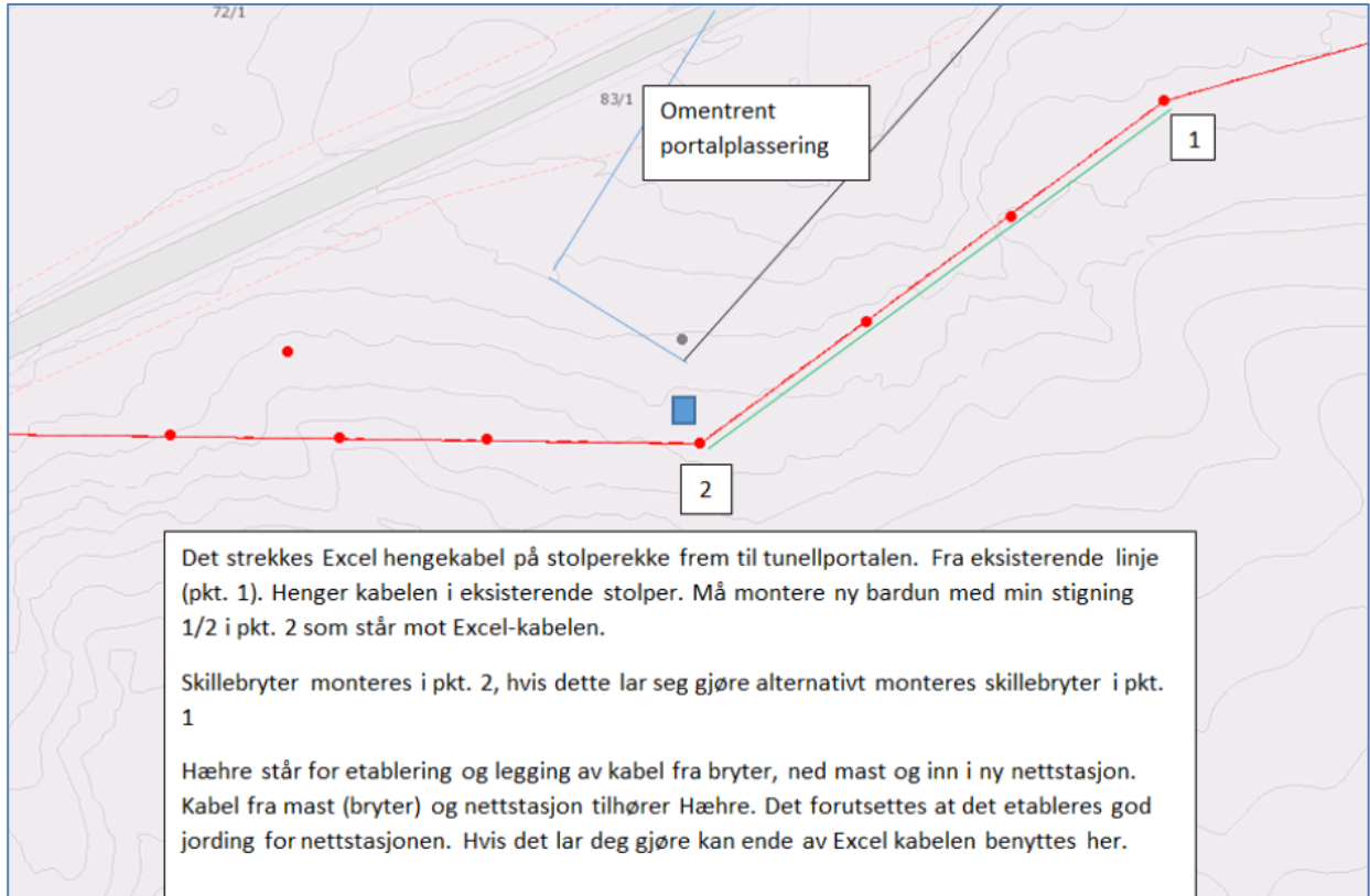
Figur 1: Skisse over område der ny container skal plasseres. Blå firkant markerer plassering av container, grønn strek viser ny 22 kV hengekabel som bygges under områdekonsesjonen til Nordlandsnett, blå strek viser omtrentlig portalplassering for tunnelen og rød strek viser eksisterende 22 kV nett. Kilde: Hæhre Entreprenør AS
