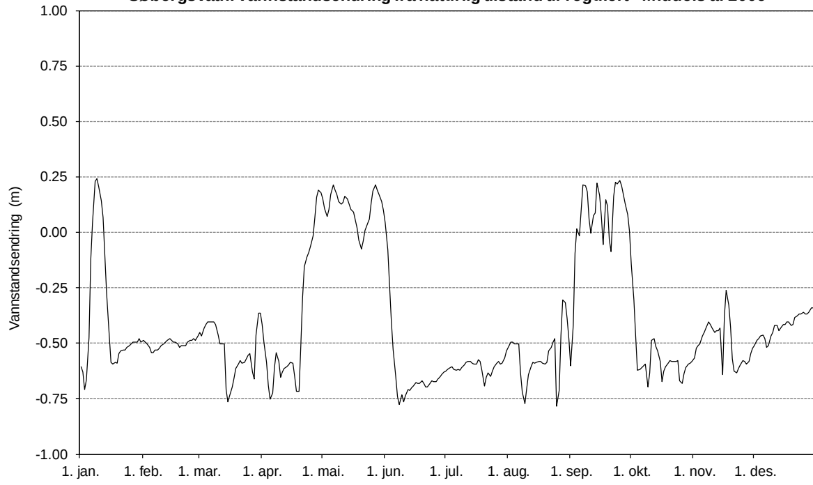
Søbergsvatn. Vannstandsending fra naturlig tilstand til regulert - Middels år 2009
