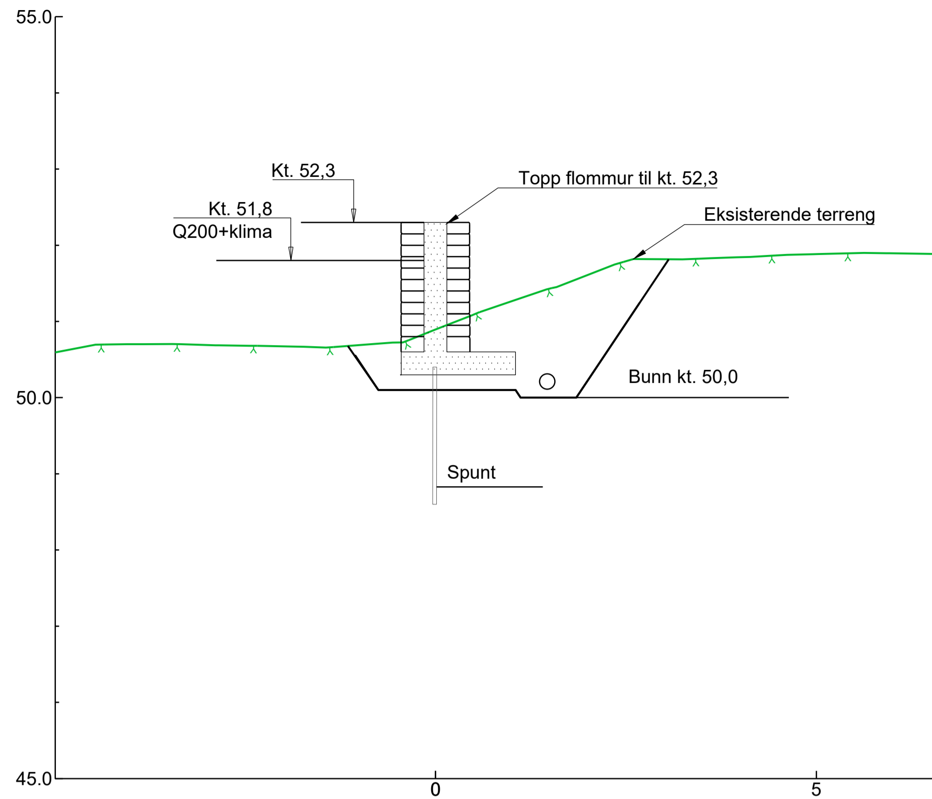
SNITT A-A Lekkemoen 1:50
