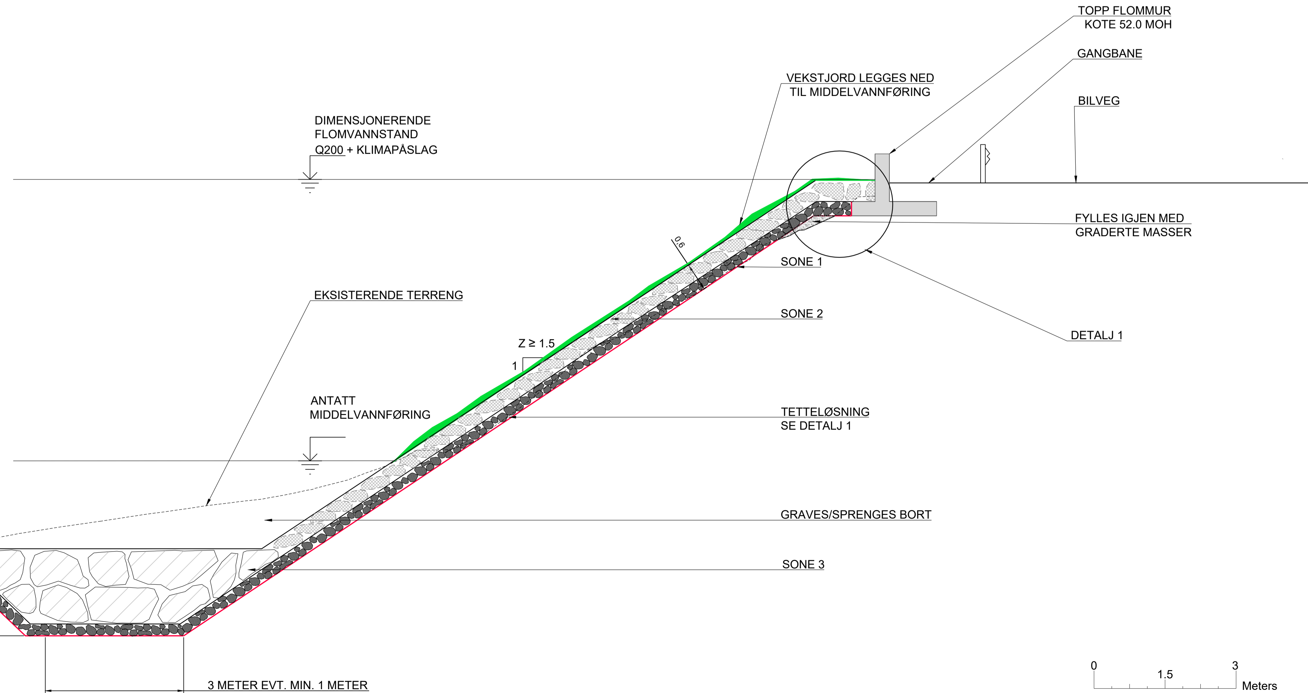
SNITT E SIKRING MED FLOMMUR GJENDESVEIEN 1:50
