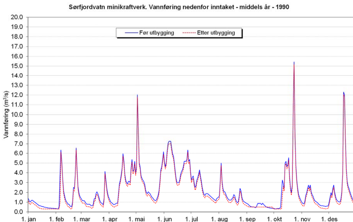
Figur 3-7. Vannføring i Sørfjordelva like nedstrøms utløpet fra Sørfjordvatnet før og etter realisering av tiltaket i et middels år.
