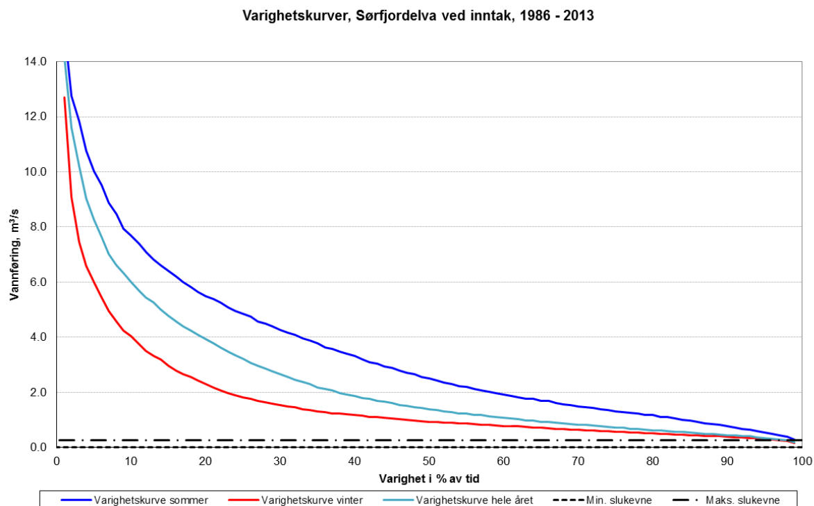
Figur 20. Varighetskurve, kurve for sommer, vinter og hele året.
