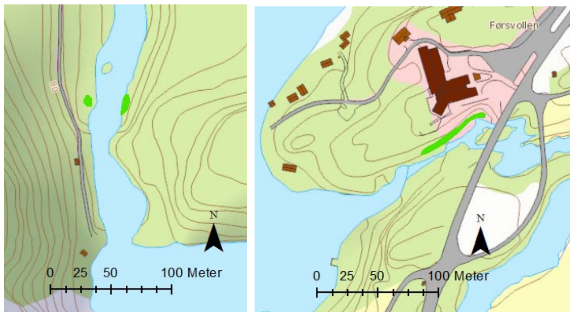
Figur 3-6 Fosseenger/-sprutsoner i Sørkjølva (grønne polygon). Til venstre: Ca. ved kote 70, like nedstrøms Sørkjølvatnet. Svært viktig (A-verdi). Til høyre: Ved Baggfossen like nedstrøms E6. Viktig (B-verdi).
