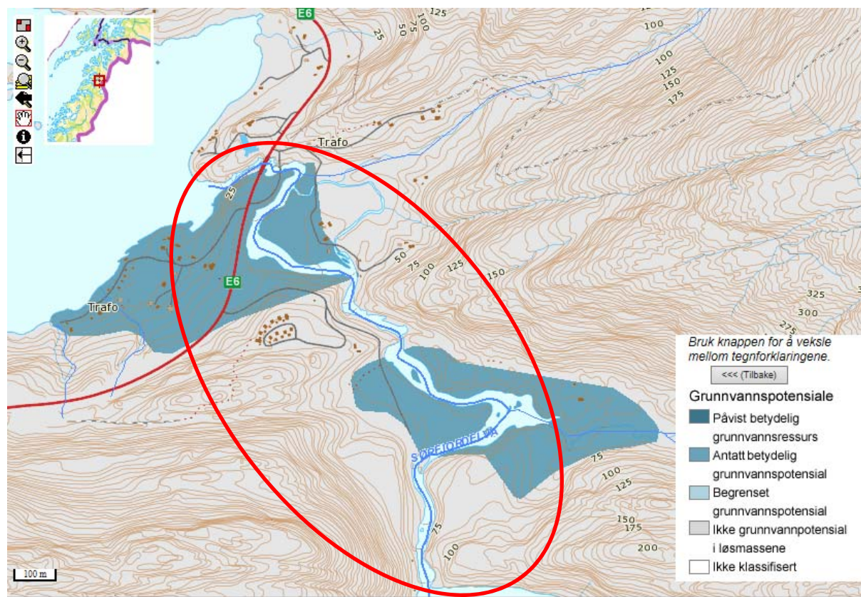
Figur 3-1 Kartutsnitt fra grunnvannsdatabasen GRANADA [3]. Berørt strekning i Sørfjordelva er markert med rødt.
