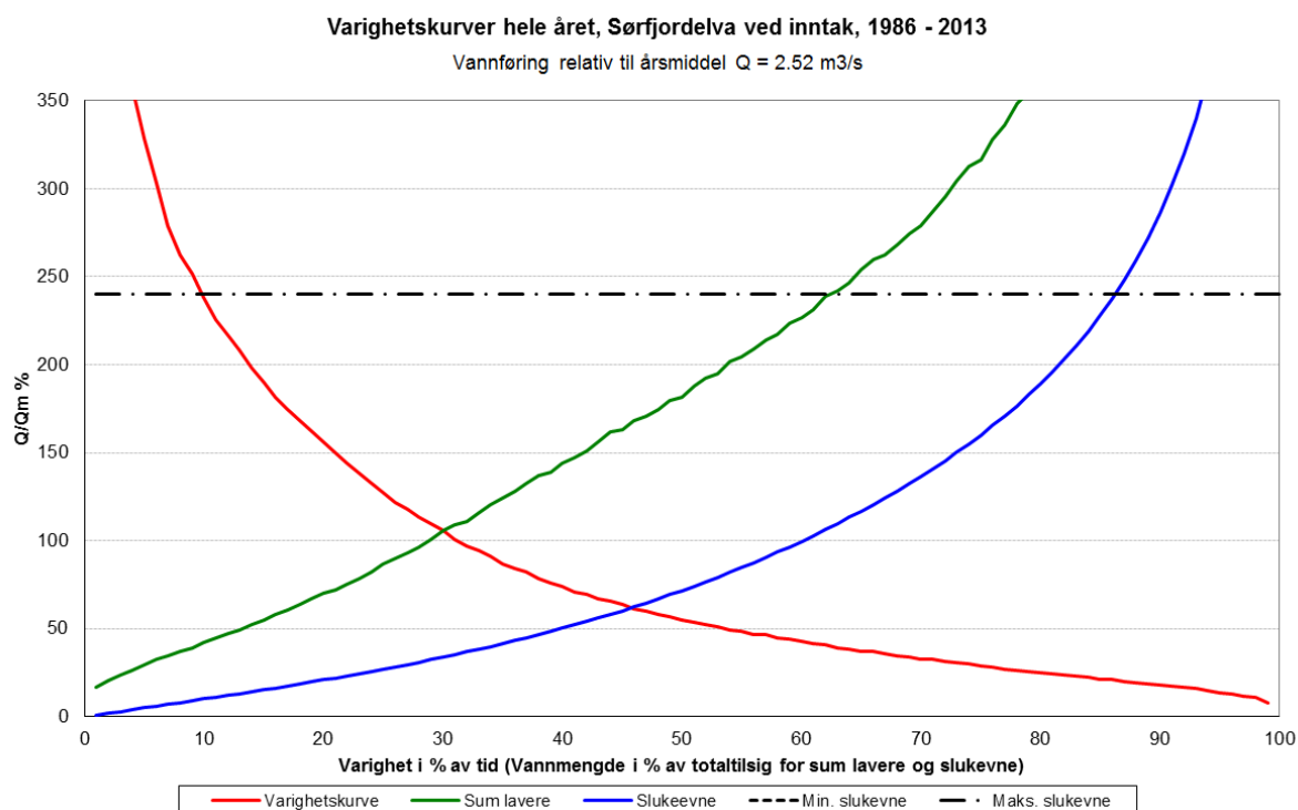
Figur 21. Varighetskurve, kurve for flomtap og for tap av vann i lavvannsperioden (år).
