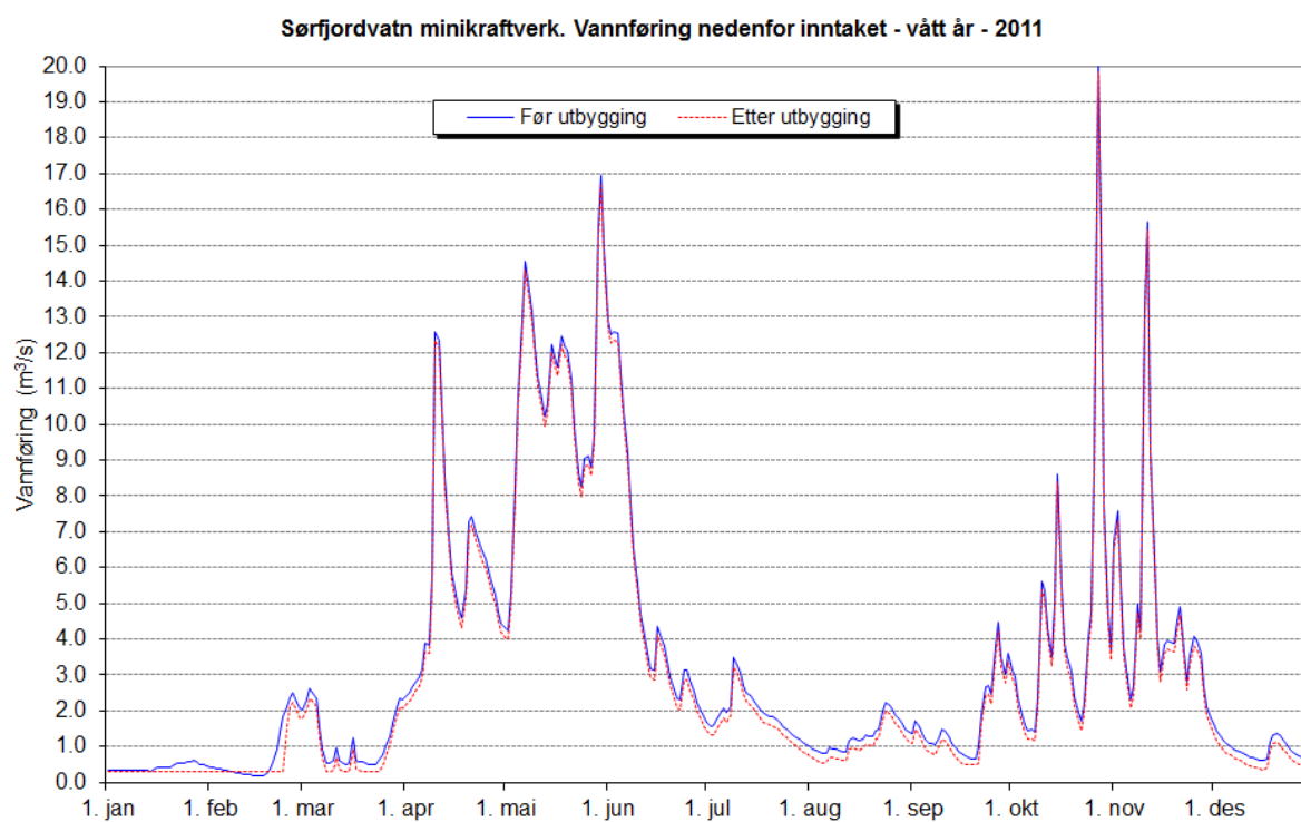
Figur 10. Plott som viser vannføringsvariasjoner i et vått (2011) år (før og etter utbygging). 21
