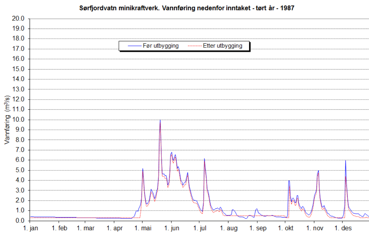
Figur 6. Plott som viser vannføringsvariasjoner i et tørt (1987) år (før og etter utbygging). 17
