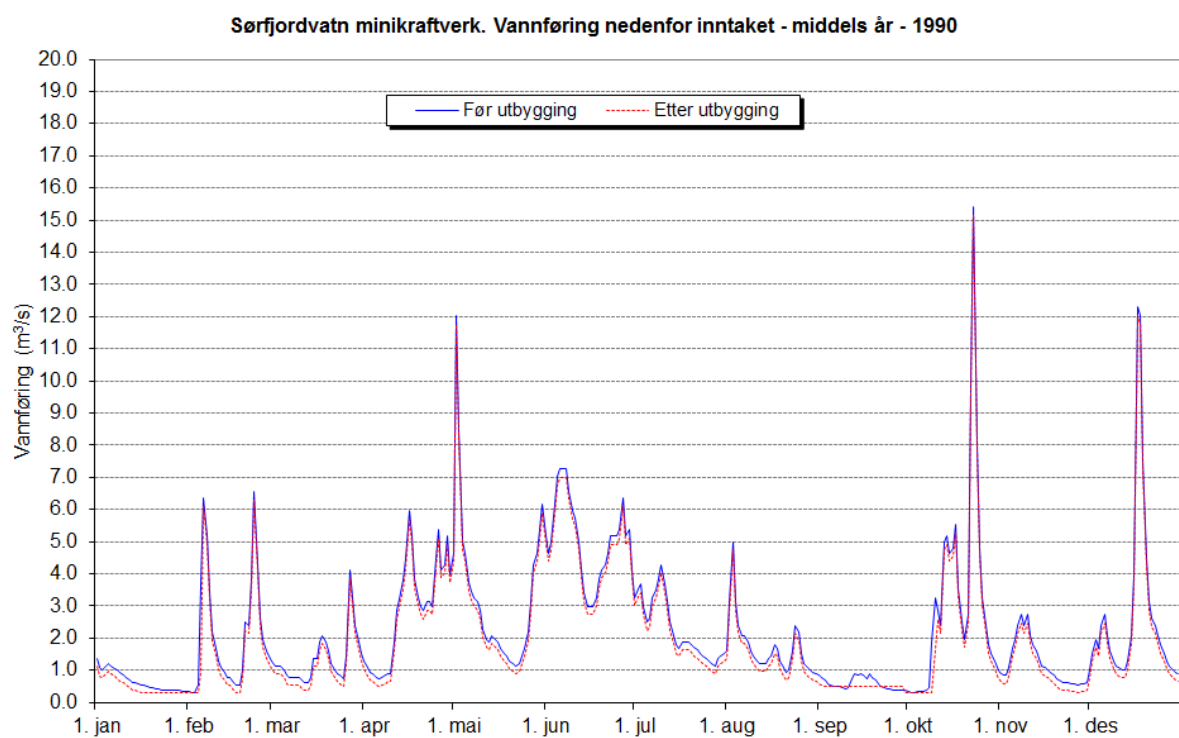
Figur 8. Plott som viser vannføringsvariasjoner i et middels (1990) år (før og etter utbygging). 19
