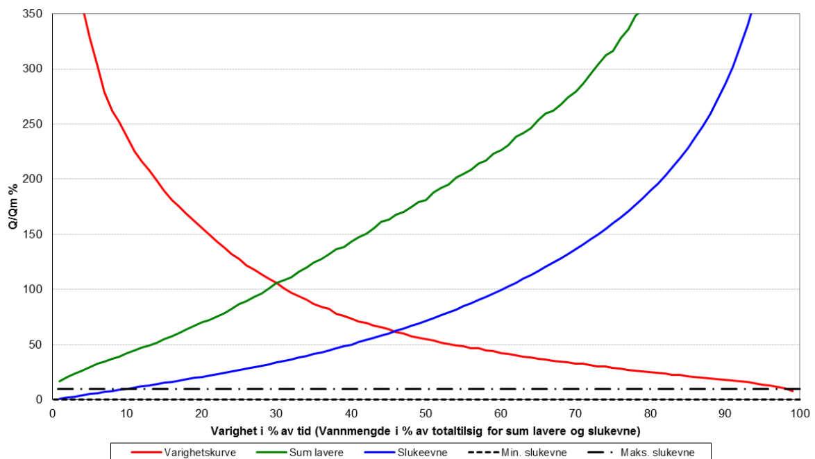
Figur 14. Varighetskurve, kurve for flomtap og for tap av vann i lavvannsperioden (år).
