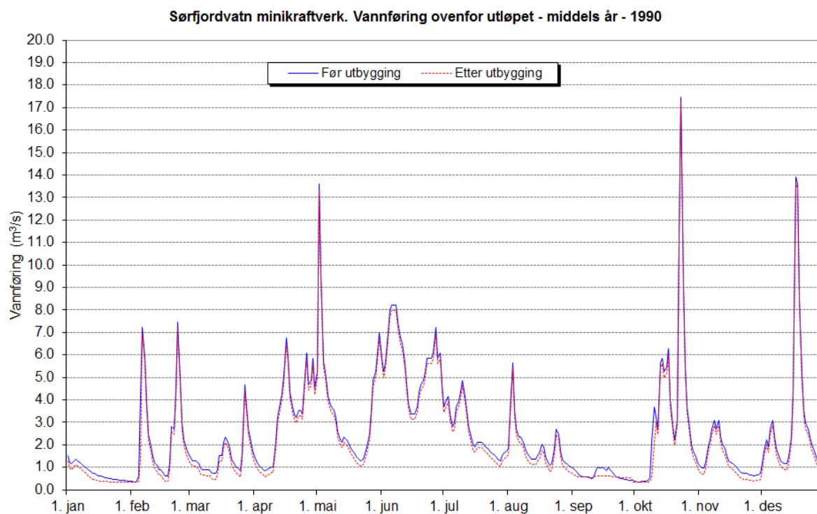
Figur 9. Plott som viser vannføringsvariasjoner i et middels (1990) år (før og etter utbygging). 20
