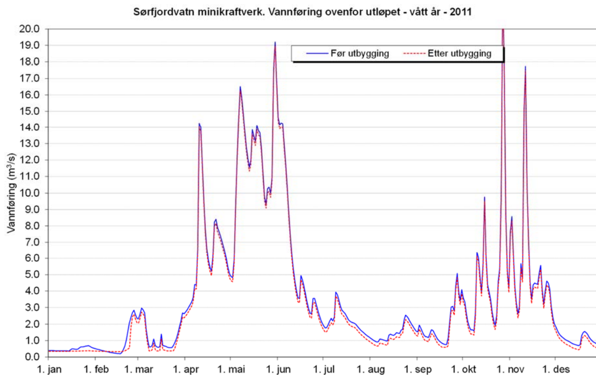
Figur 11. Plott som viser vannføringsvariasjoner i et vått (2011) år (før og etter utbygging). 22
