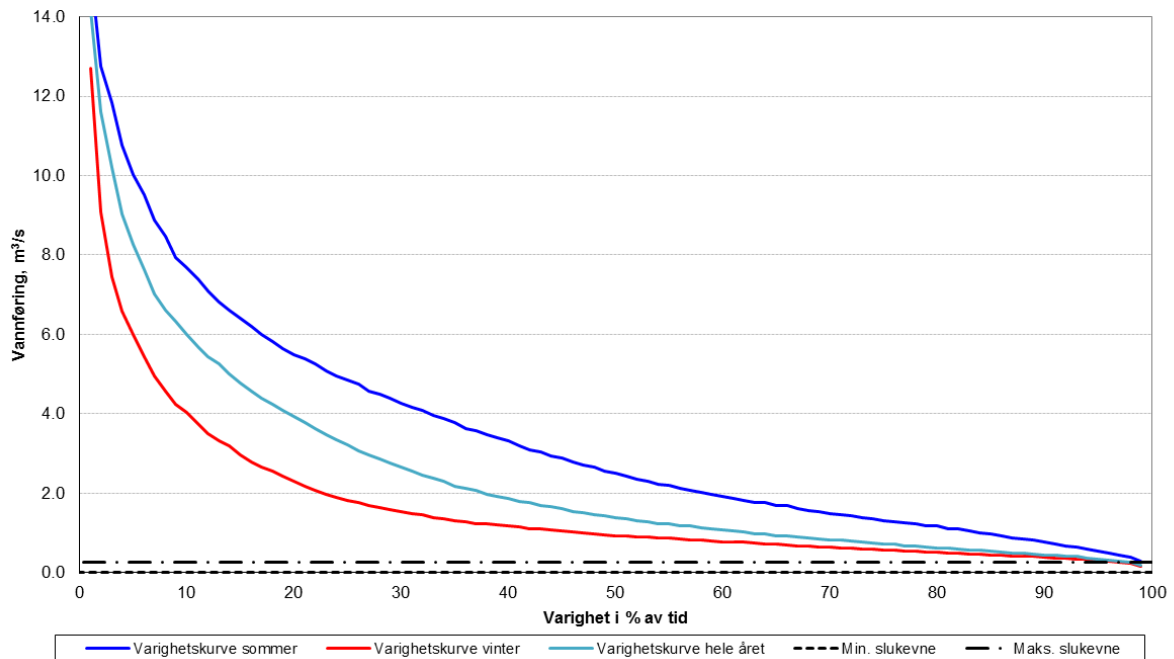
Varighetskurver, Sørfjordelva ved inntak, 1986 - 2013
