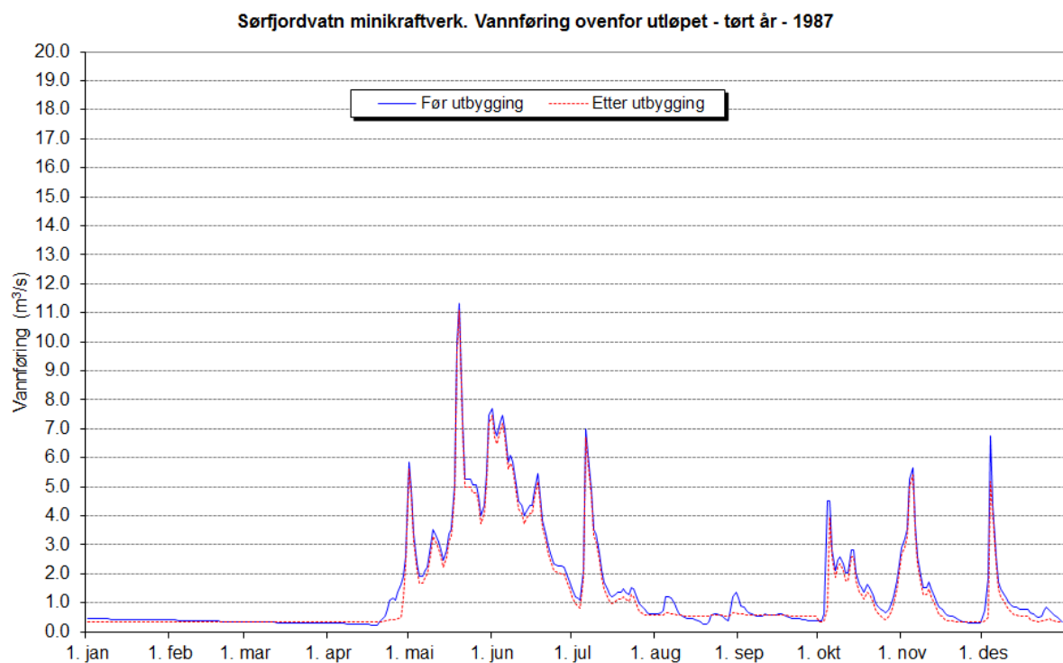
Figur 7. Plott som viser vannføringsvariasjoner i et tørt (1987) år (før og etter utbygging). 18
