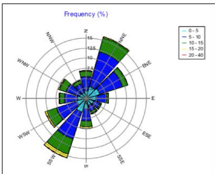
Figur 6-1. Vindrose som viser fremherskende vindretning i planområdet. Kilde: Kjeller Vindteknikk.
