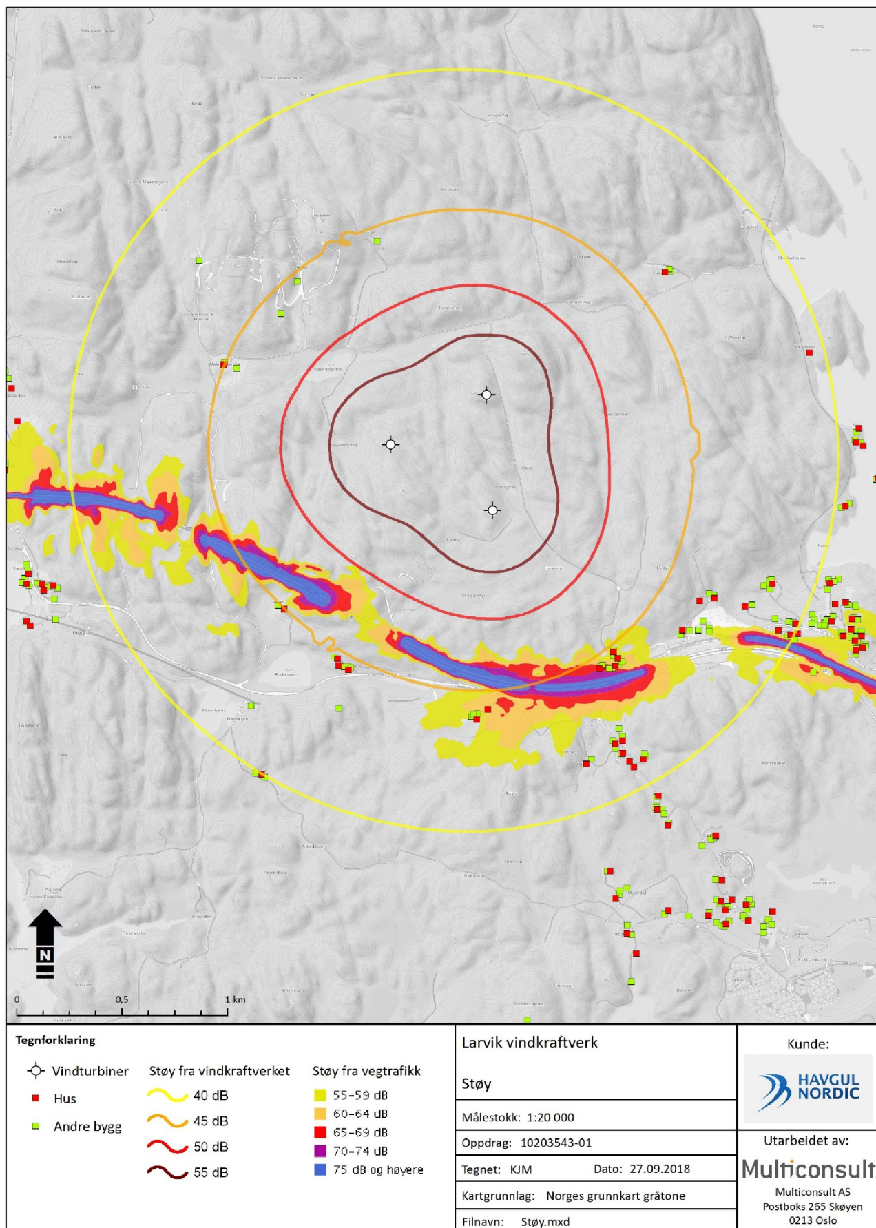
Figur 7-30. Beregnet støynivå (dB) fra vindkraftverket og vegtrafikk. Kilde: Kjeller Vindteknikk og Statens vegvesen.
