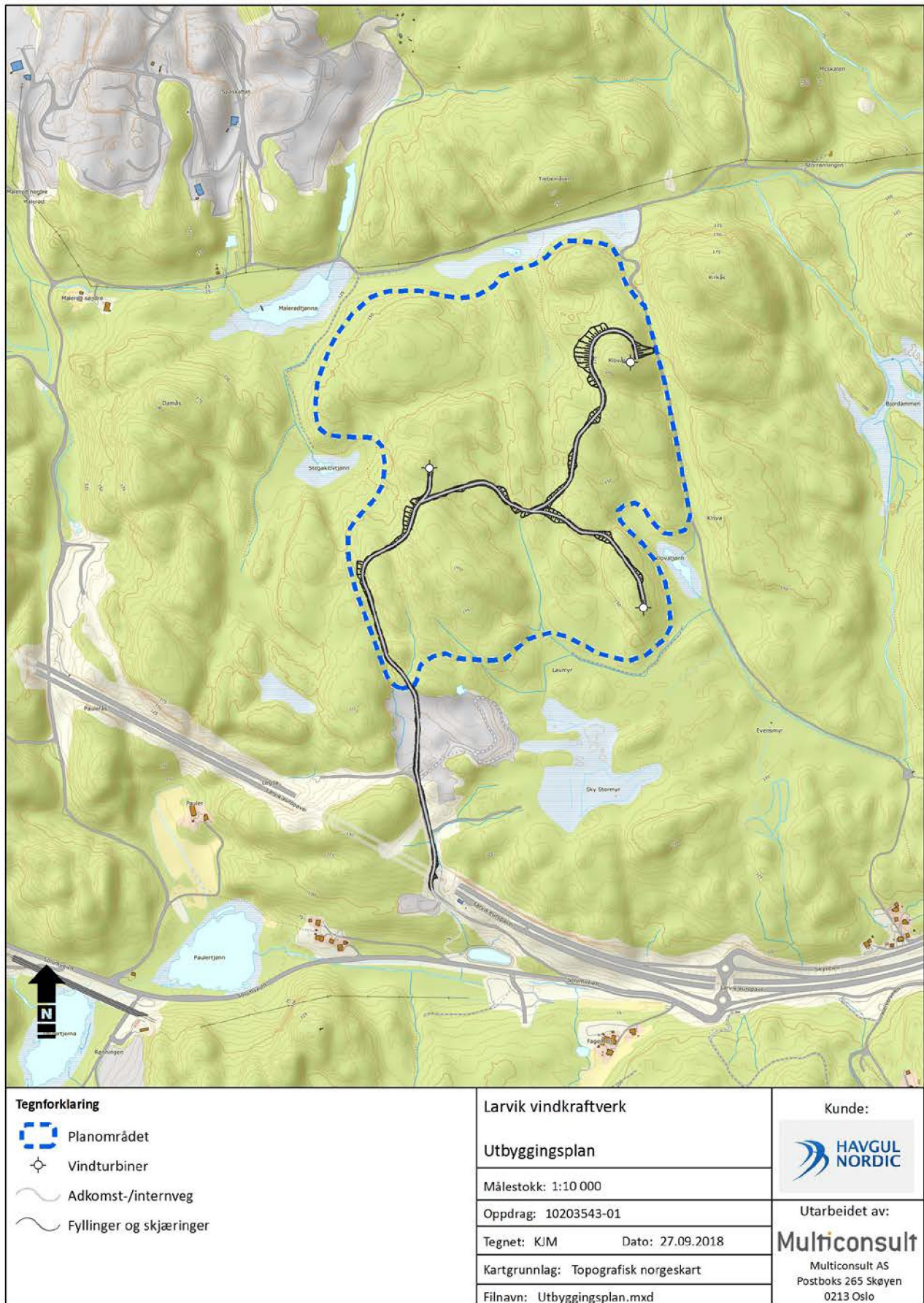
Figur 1-2. Oversikt over Larvik vindkraftverk med tilhørende infrastruktur.
