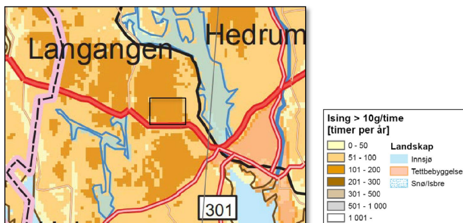
Figur 7-33. Isingskart for området (Kjeller Vindteknikk, 2009).
