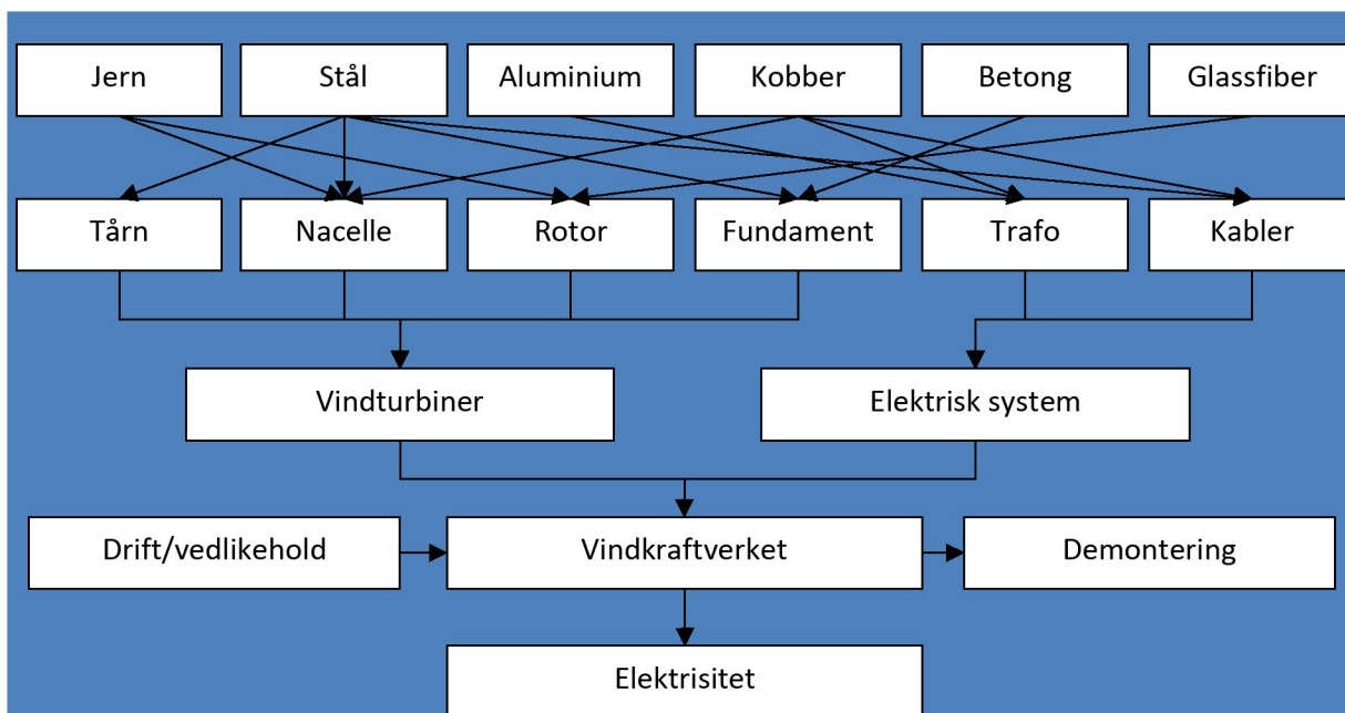
Figur 7-34. Forenklet verdikjede for et vindkraftverk.
