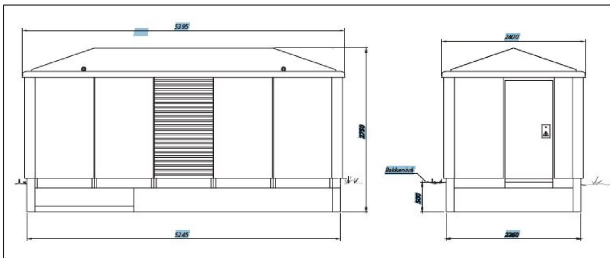
Figur 5-4. Skisse for planlagt kiosk.
