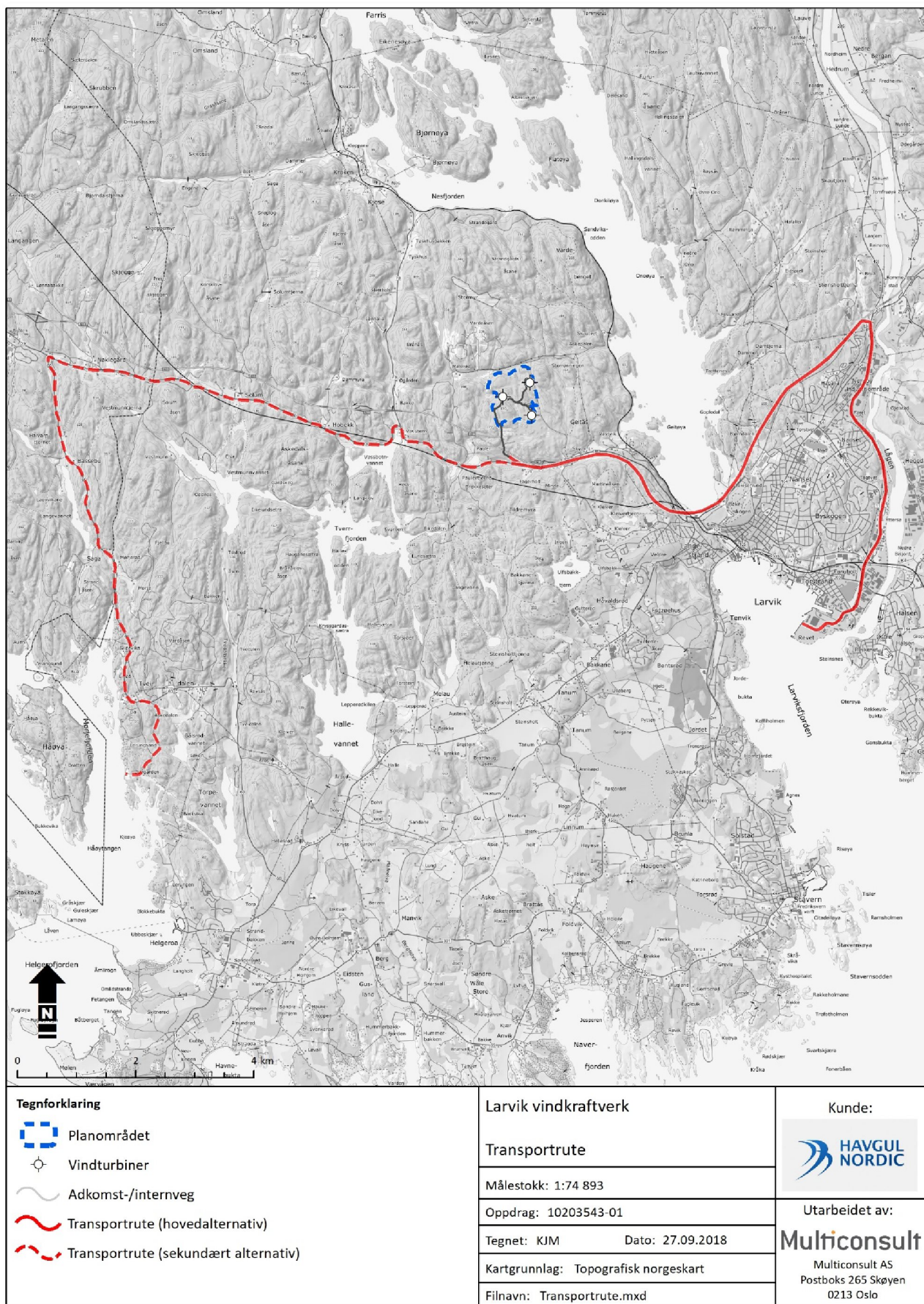
Figur 5-2. Transportrute mellom havna i Larvik eller ved Svartebukt og planområdet, samt internveier i vindkraftverket.
