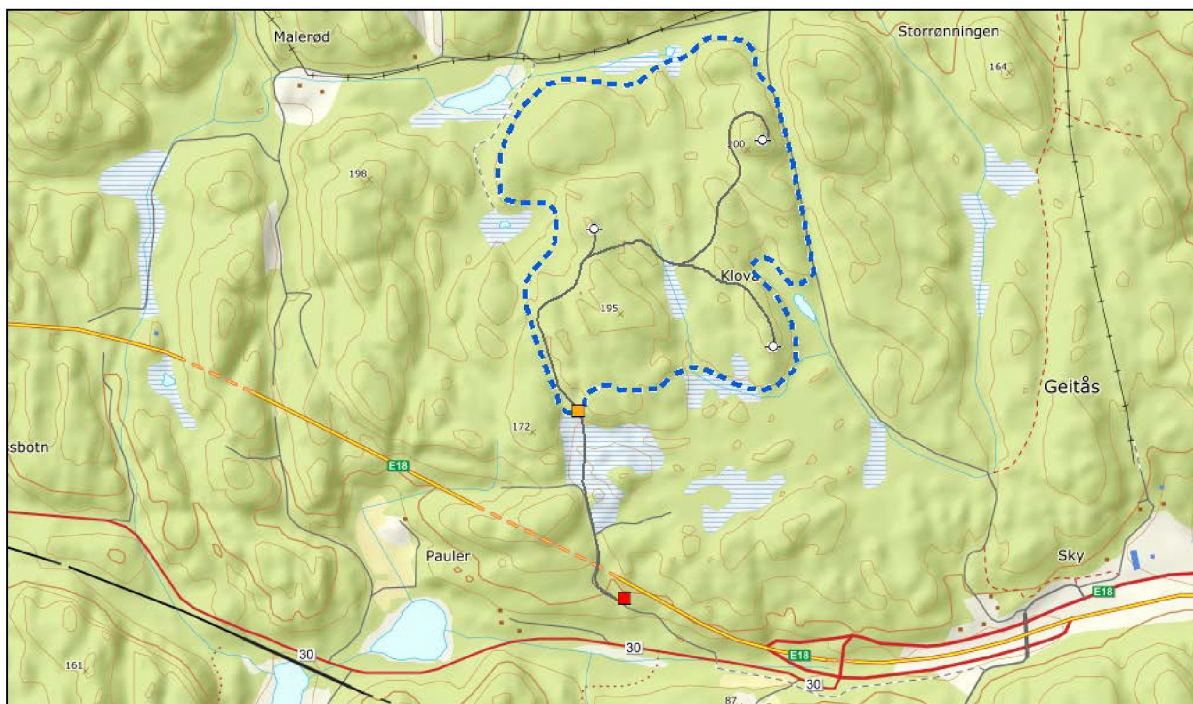
Figur 5-3. Planlagt påkoblingspunkt (nettstasjon) ved E18 er merket med rød firkant. Ny kiosk (se beskrivelse under) er angitt med oransje firkant. Jordkabelen legges i grøft langs vegskulder på adkomst-/internvegene.
