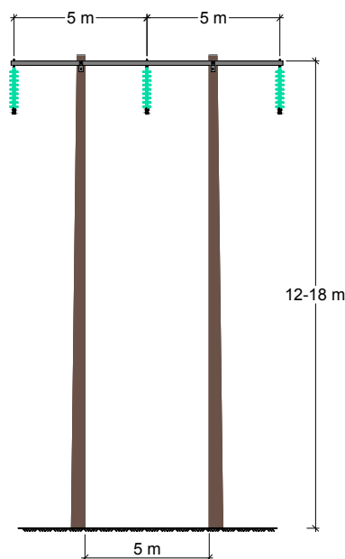
a) Portalmast med trestolper, ståltravers og glassisolatorer
