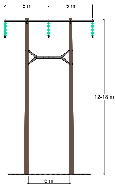
b) Som a) men, forsterket med stålriegel
