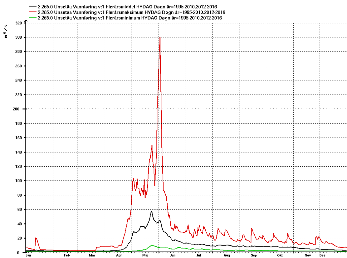
Plott av vannføring Unsetåa i perioden 1995 til 2016
