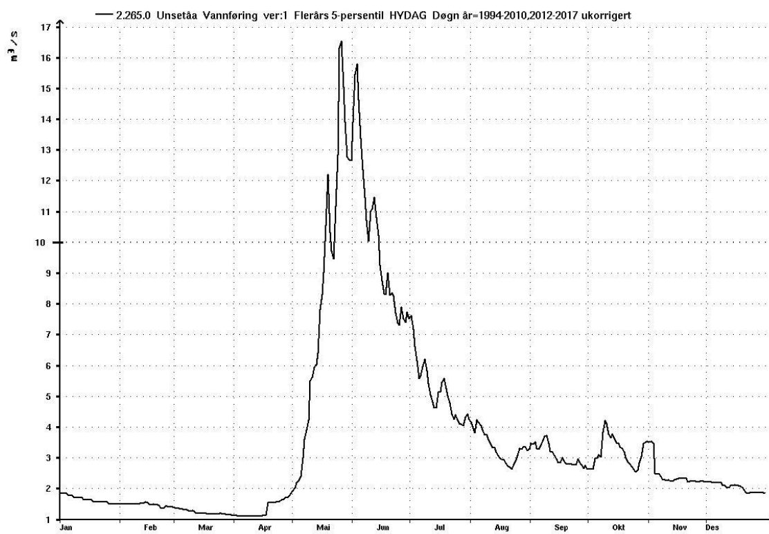
Plott av 5-persentil Unsetåa i perioden 1994 til 2017
