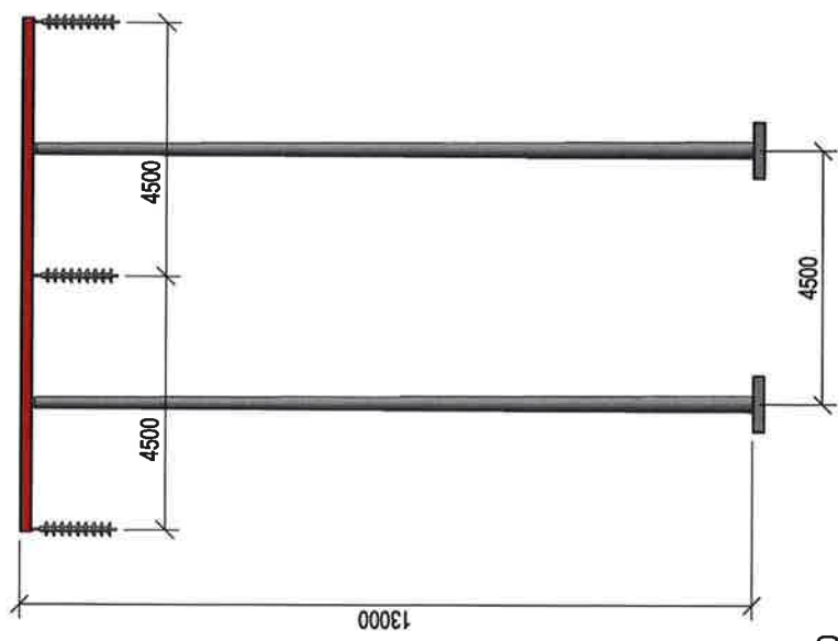
Snitt 1 : 100
