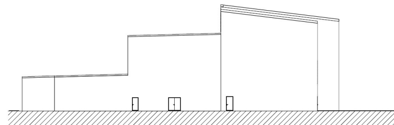
NORD / NORTH 1 : 200
