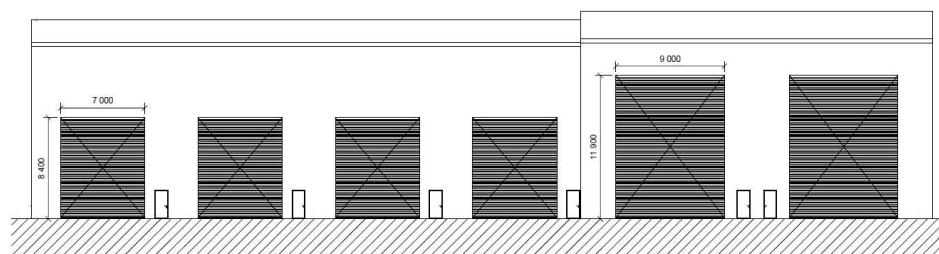
VEST / WEST 1 : 200
