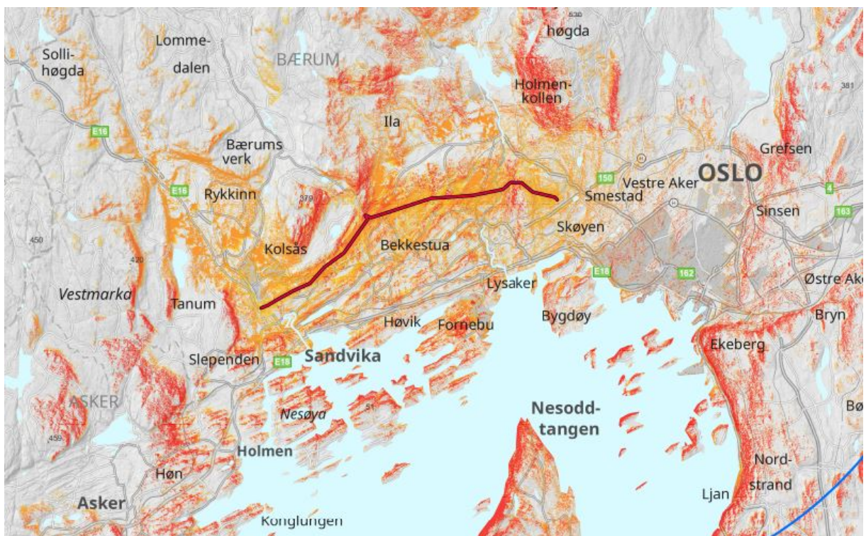
Figur 5-48 Utsnitt av synlighetskart som viser overordnet situasjon for alternativ med luftspenn. Kilde: Sweco Norge AS.
