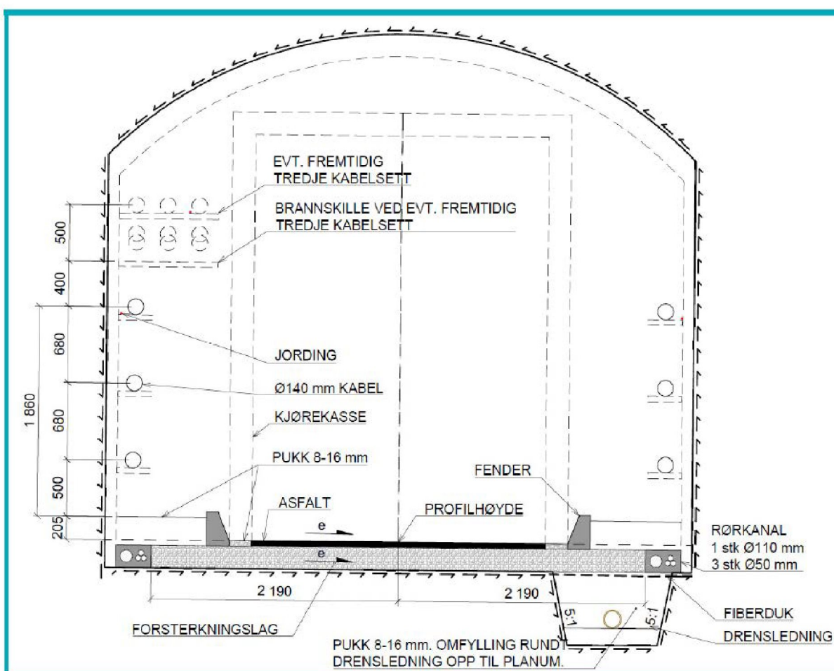
Figur 1-1. Skisse av kabelsett. Kilde: Norconsult 2017.
