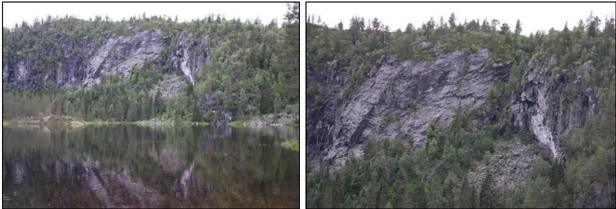
Figur 12. Naturtypen sørvendt berg og rasmark (B01) opptrer i Svartetjørnheii, som ligger sørvest for inntaksmagasinet Svartetjørn. Bare nordlige del av naturtypelokaliteten, dvs. høyre del av hvert bilde, vender mot sør-sørøst. Foto: Ole Kristian Spikkeland.
