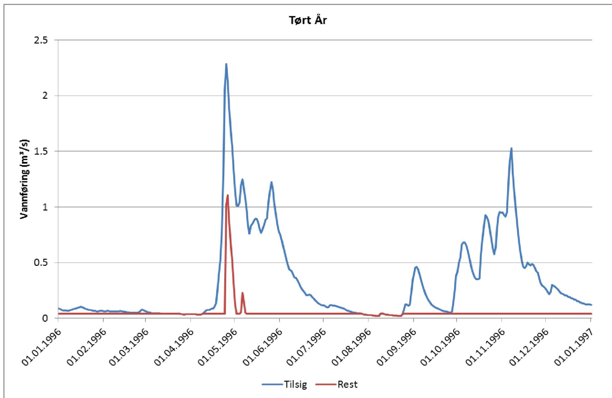
Figur 28. Vannføringsvariasjoner i Kvernåni i et tørt (1996) år før og etter utbygging. Maksimal slukeevne er 1,02 m 3 /s (kilde: Multiconsult AS).
