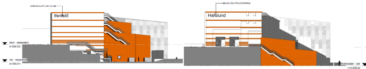
Figur 3: Fasade øst
