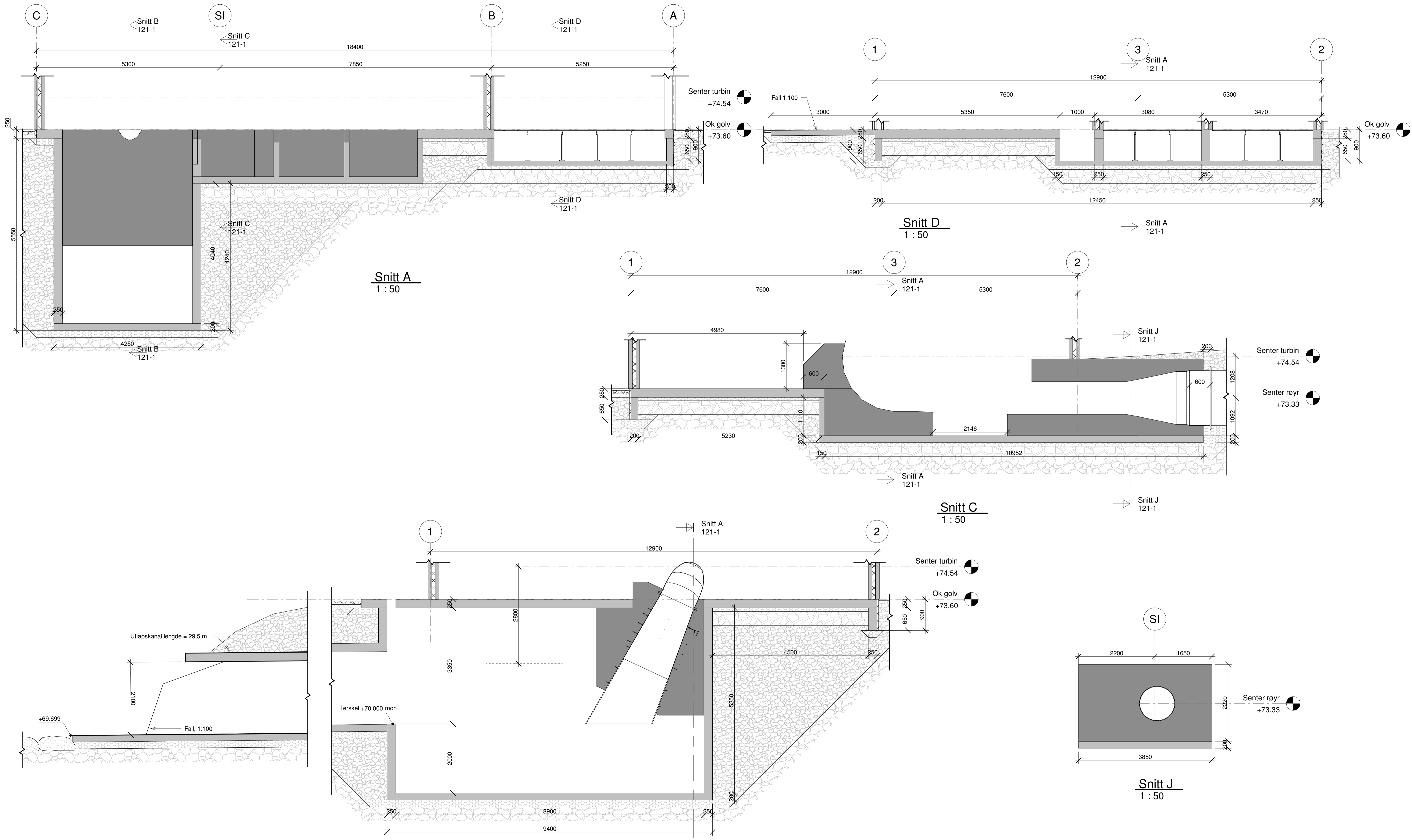
Snitt B 1 : 50
