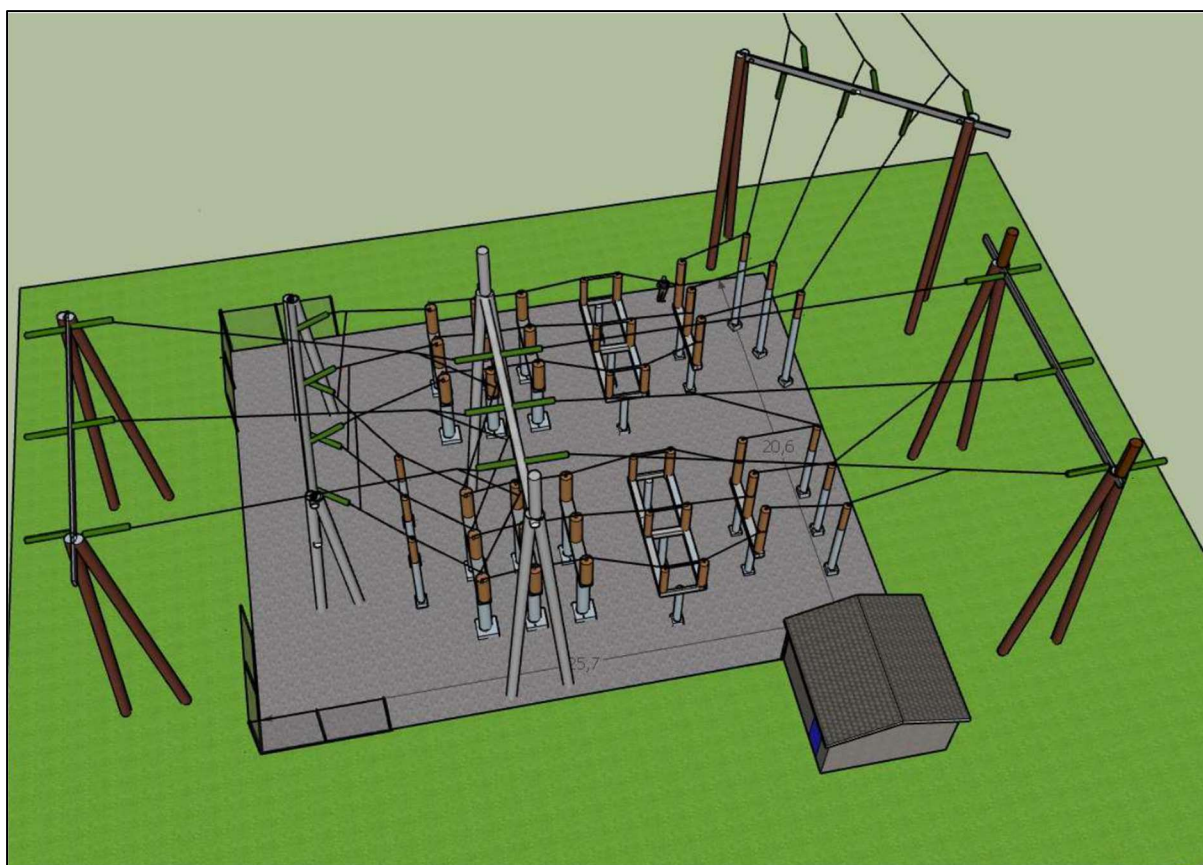
Sveinsøystølen koblingsanlegg – skisse med kontrollhus/nettstasjon
