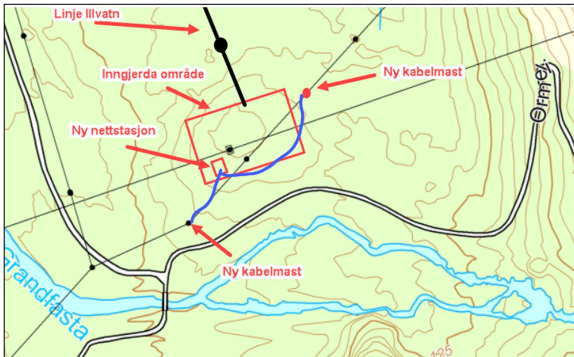
Sveinsøystølen koblingsanlegg – inngjerdet areal, nettstasjon og 22 kV jordkabel
